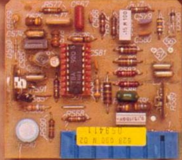
Zeilengenerator
