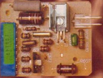
ZF-Verstärker
