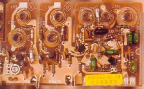
Bild-Kipp-Modul
