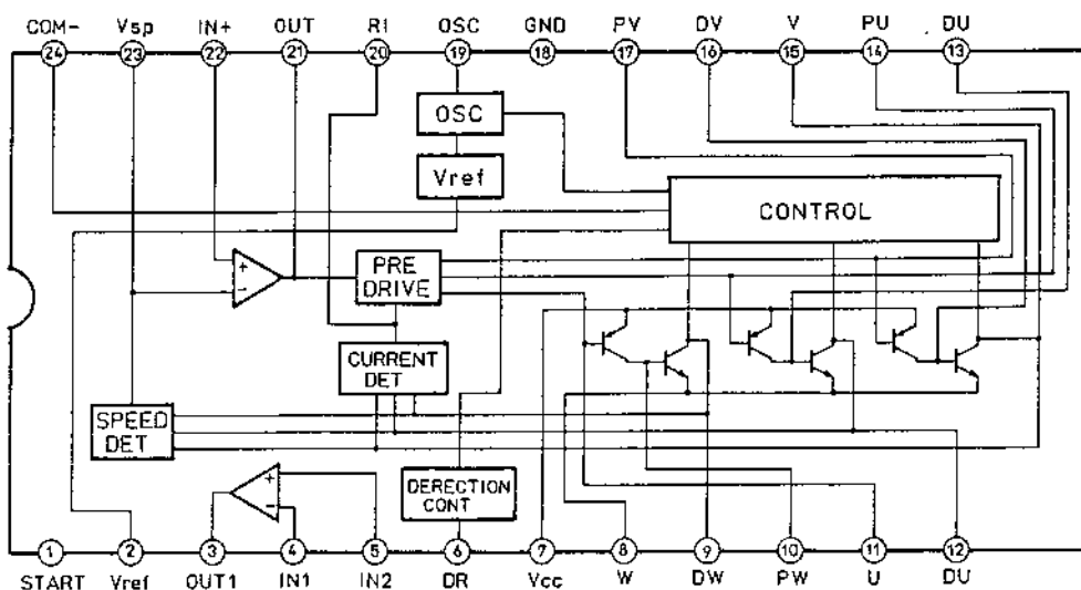
IC601 LB1672M
