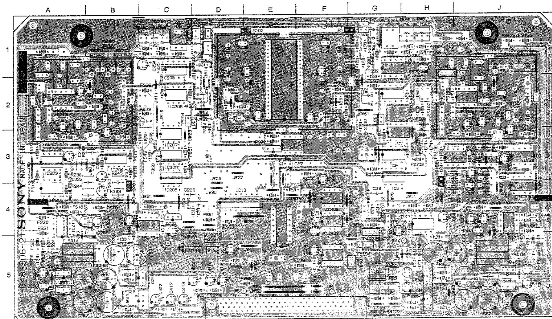
AP-31A 1-648-906-21 A SIDE
