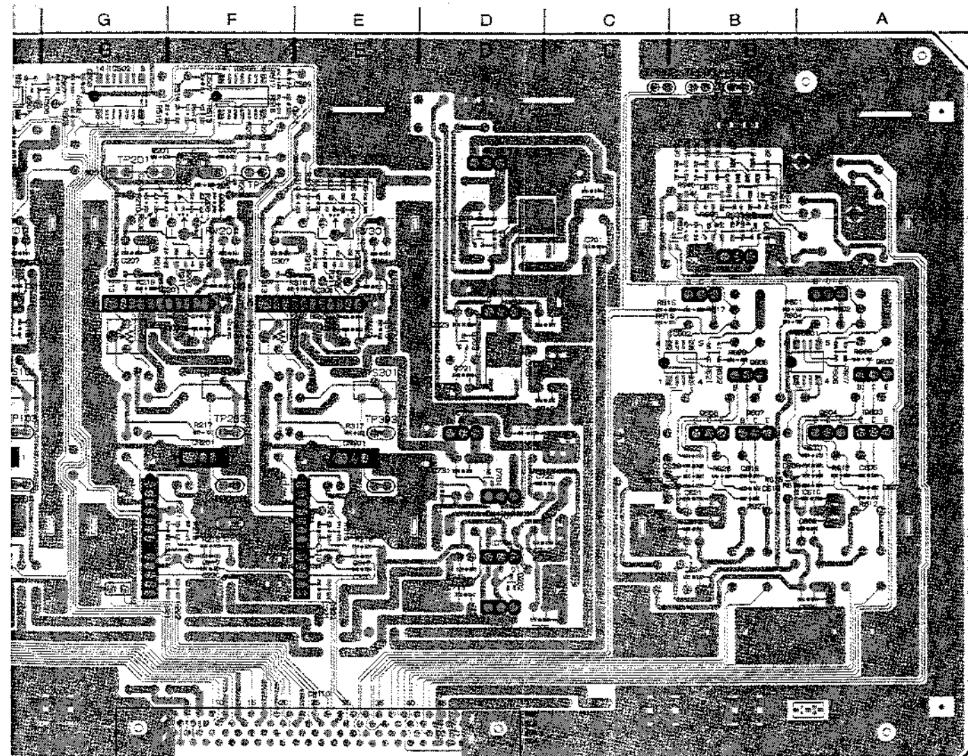
RP-70 1-648-904-11 B SIDE
