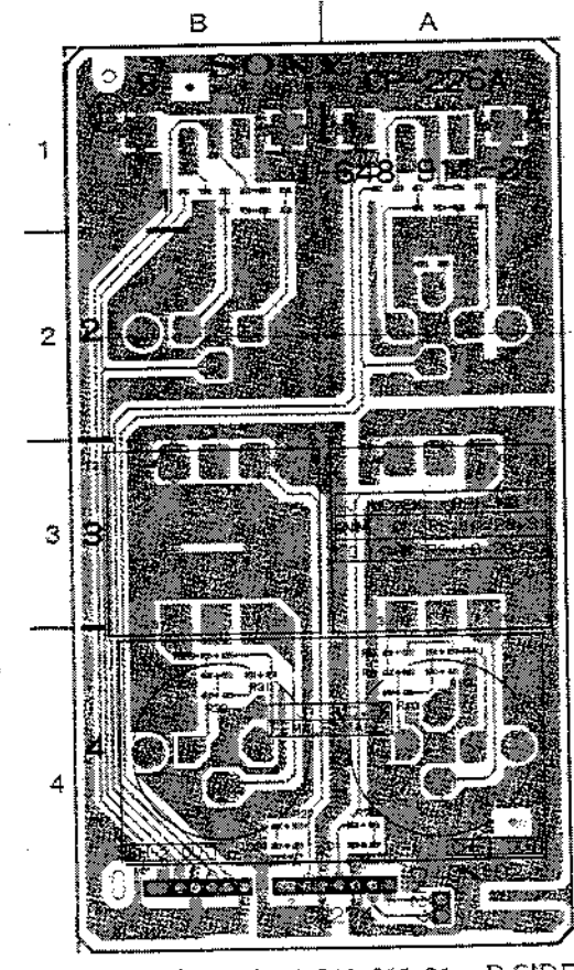
CP-226A/226AJ 1-648-911-21 B SIDE
