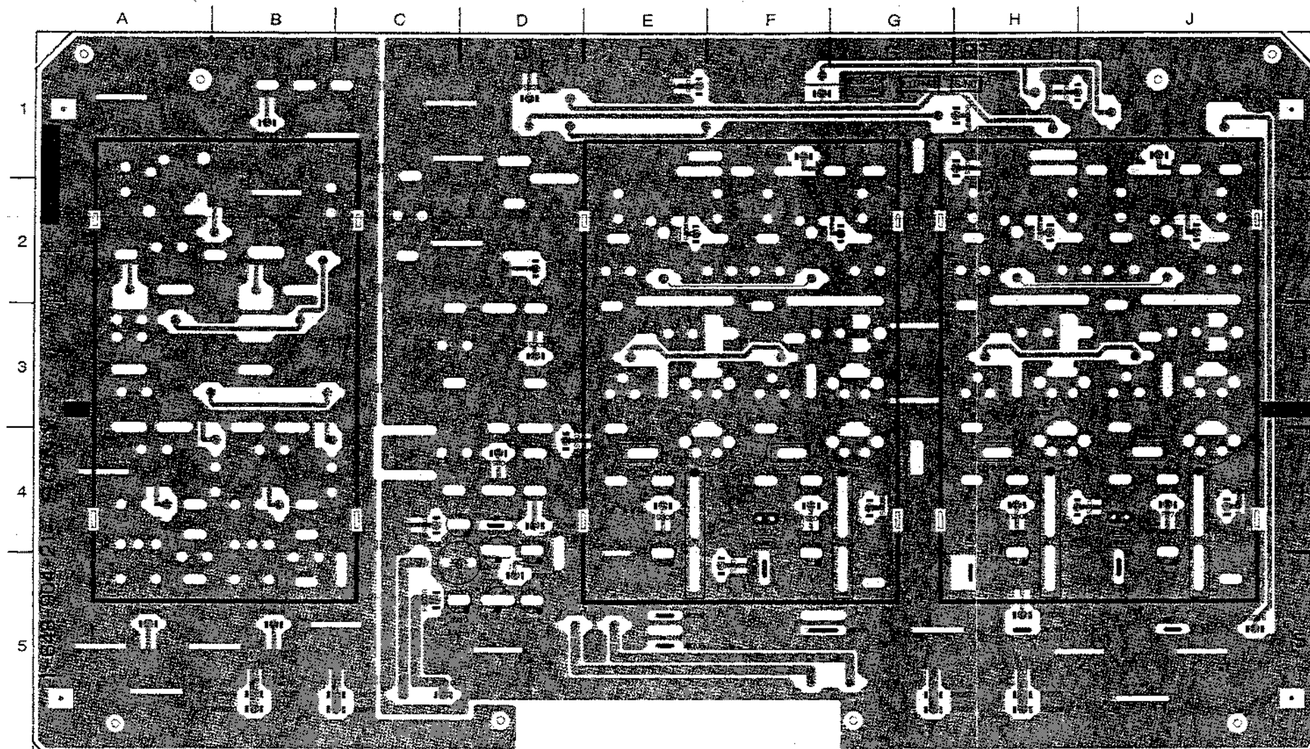
RP-70A 1-648-904-21 A SIDE
