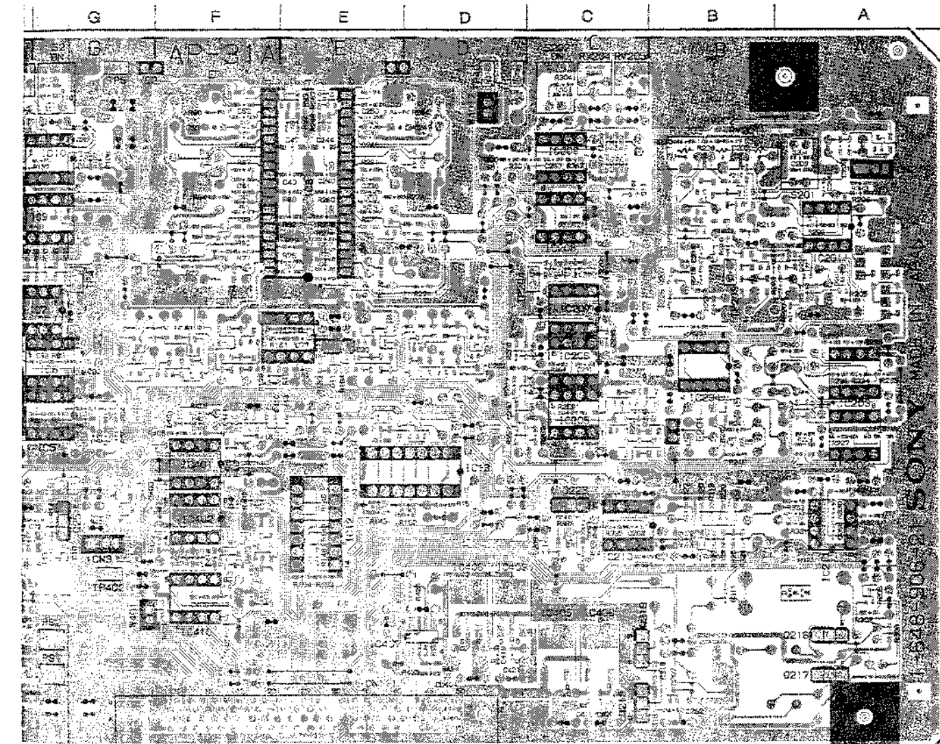
AP-31A 1-648-906-21 B SIDE
