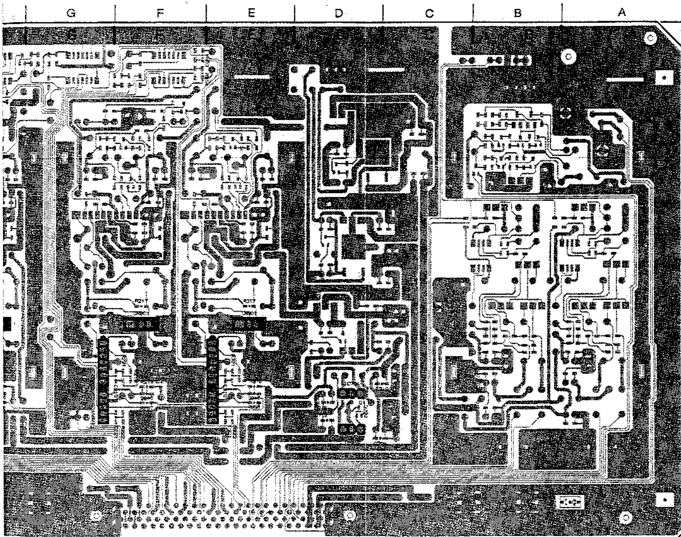
RP-70A 1-648-904-21 B SIDE
