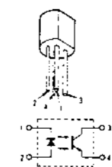
NJL5141E-AA
