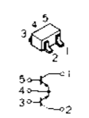
NJL5141E-AA
