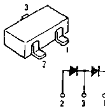
CL-170PG-CD-T
