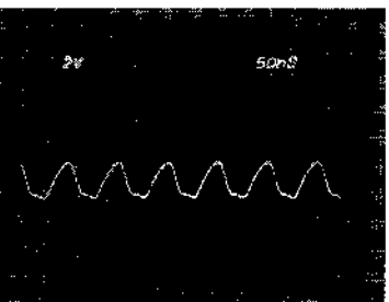
⑩ IC304⑬ } 2.4Vp-p TP311
