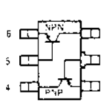
XN4315
