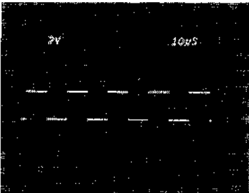
⑥ IC304⑪ } 2.7Vp-p TP310
