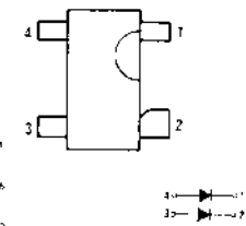
MA713
