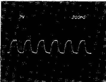
④ IC304⑫ } 3.0Vp-p TP308 (XBCK)
