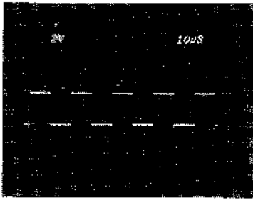
① TP309 (LRCK) 3.1Vp-p
