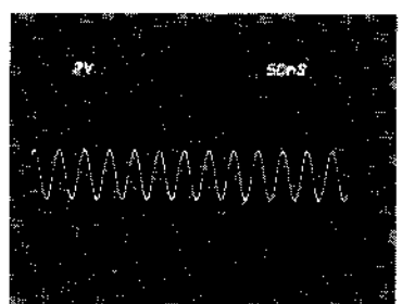
⑥⑤ IC508⑥⑤ 3.2Vp-p
