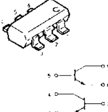
XN4504
