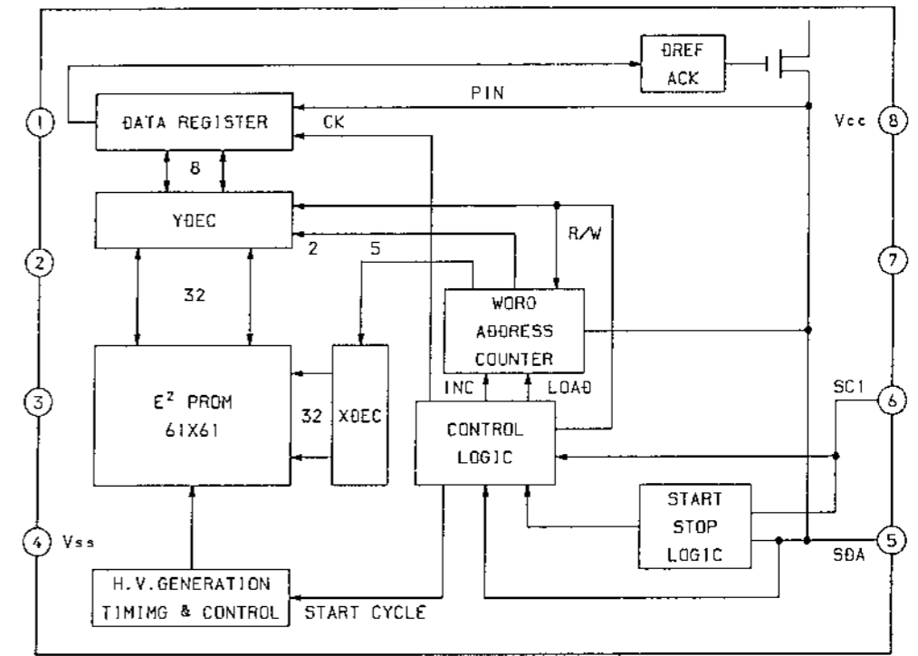
IC902 X24C01P-S
