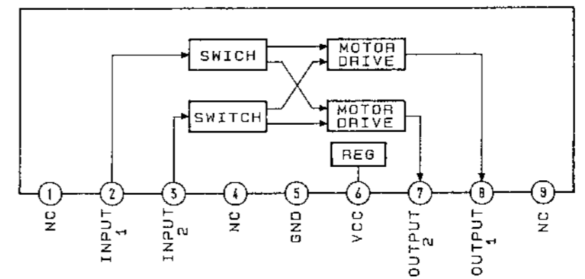
IC903 BA6208
