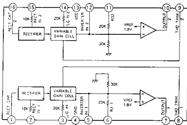
IC280, 281 NE571N-A
