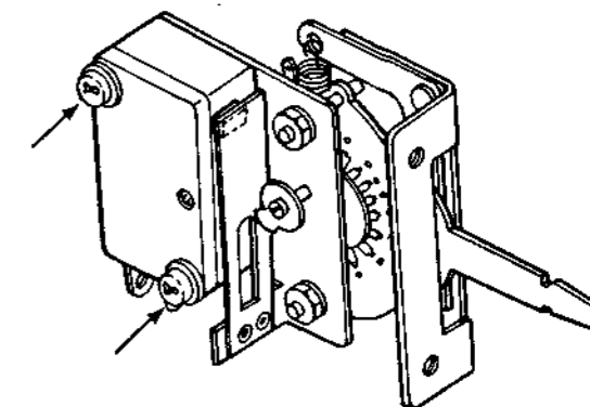
Fig. 2-7. Microswitch Replacement
