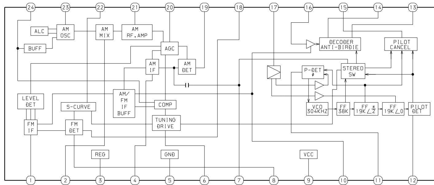
IC, LA1845N-A
