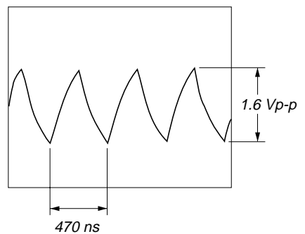
① IC711 ⑥ (OSCI)
