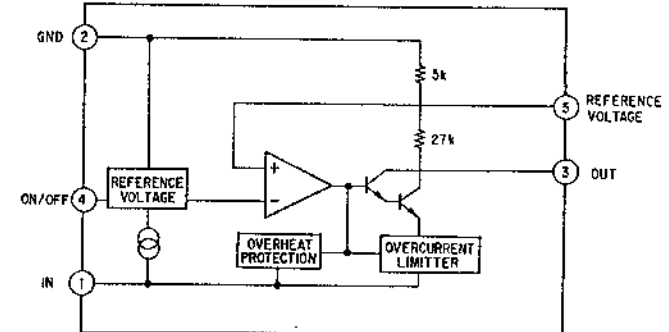
IC908 M5293L
