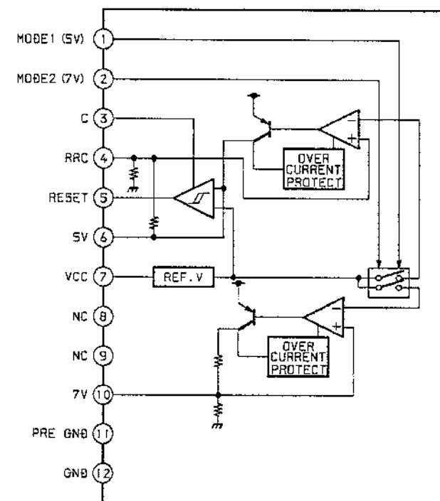
IC902 BA3963
