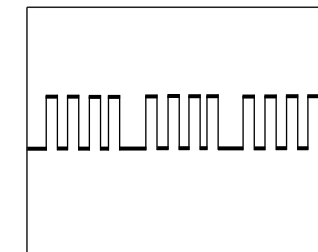
③ IC901 ② (LINE : RGB mode)
