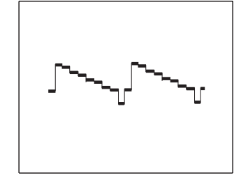
④ IC901 ② (LINE : S VIDEO mode)
