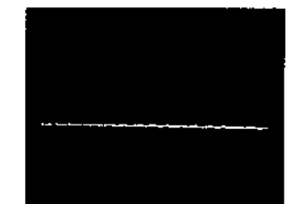
7 IC702 1pin (DATA) 6.4Vp-p, 0.3μs
