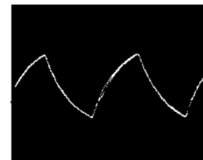
㉚ IC501 ⑩pin, IC601 ③pin (128FS) 3.4Vp-p, 50ns
