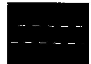
10 IC702 3pin (LRCK) 5.7Vp-p, 20μs
