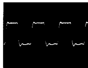
㉗ IC307 ⑤pin (F128) 6Vp-p, 50ns
