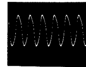
㉜ IC330 ⑩pin (XOUT) 2Vp-p, 20μs
