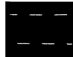
⑲ IC504 ⑦pin (LRCKI) 4Vp-p, 5μs
