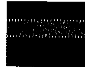
⑫ IC601 ⑩pin (1024FS) 2.4Vp-p, 50ns
