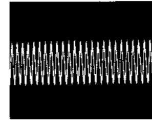
㉔ IC307 ㉒pin 1Vp-p, 49MHz
