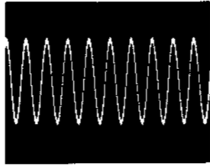
⑭ IC307 ⑭pin 3Vp-p, 18MHz
