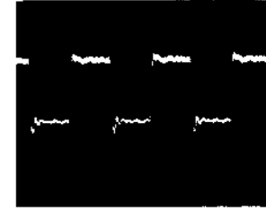
㉘ IC362 ⑩pin 7Vp-p, 0.5μs
