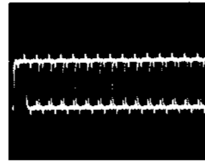
⑧ IC306 ⑧pin 5Vp-p, 0.5μs
