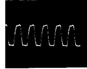
㉗ IC363 ⑧pin 6.4Vp-p, 0.1μs
