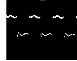
㉕ IC359 ㉑pin 5.6Vp-p, 0.5μs
