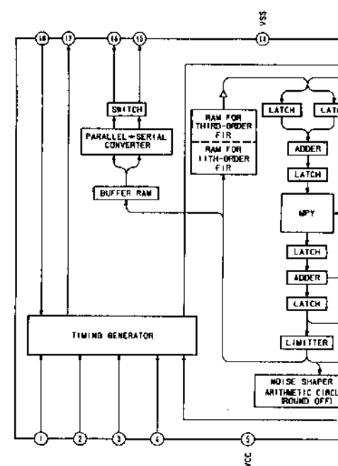
IC302 CXD2551P
