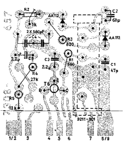
F IV, Lötseite F IV, SOLDER SIDE
