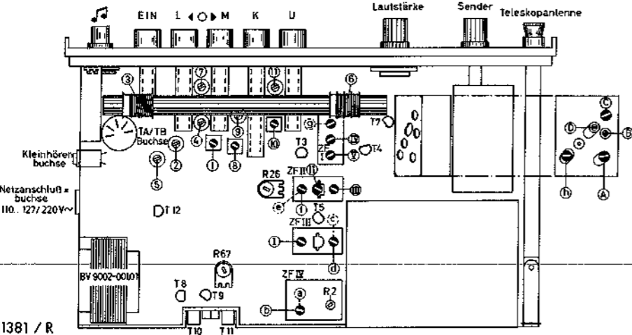
Abgleich-Lageplan ALIGNMENT SCHEME
