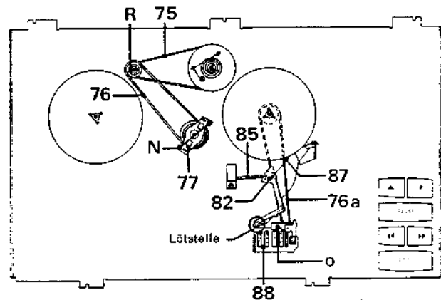
Abb. 9 Riemenwechsel
