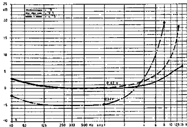
Abb. 17 Entzerrerkurve Aufnahme
