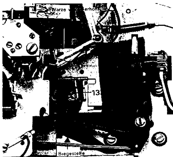
Abb. 21 Nachbiegen des Starthebels
