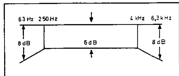
Abb. 15 Toleranzfeld nach DIN 45511 (4,75 cm/s)
