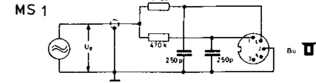
Abb. 19 Meßschaltungen
