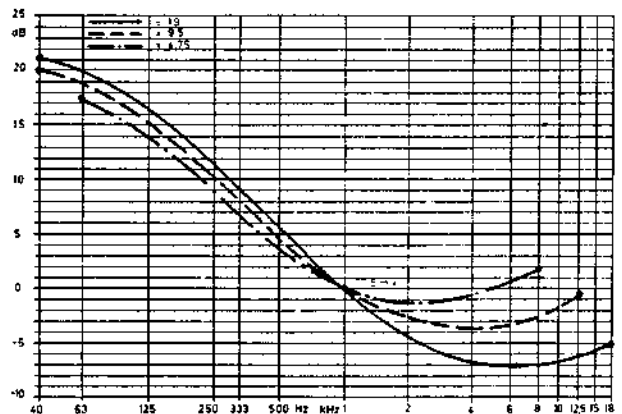
Abb. 18 Entzerrerkurve Wiedergabe
