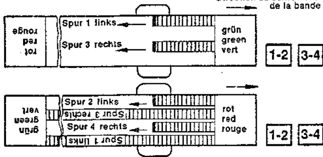
Skizze 2: Stereobetrieb Fig. 2: Stereo operation Croquis 2: Utilisation Stéréo
