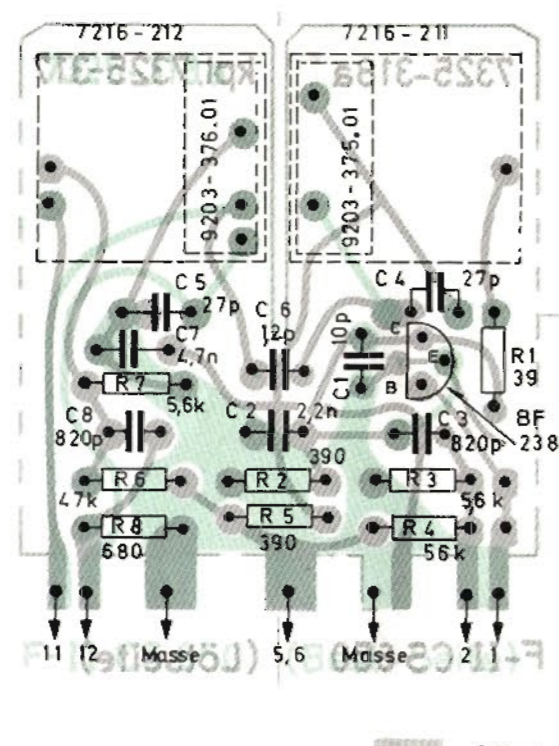
Lötseite SOLDER SIDE VUE DU COTE DES SOUDURES LATO SALDATURE
