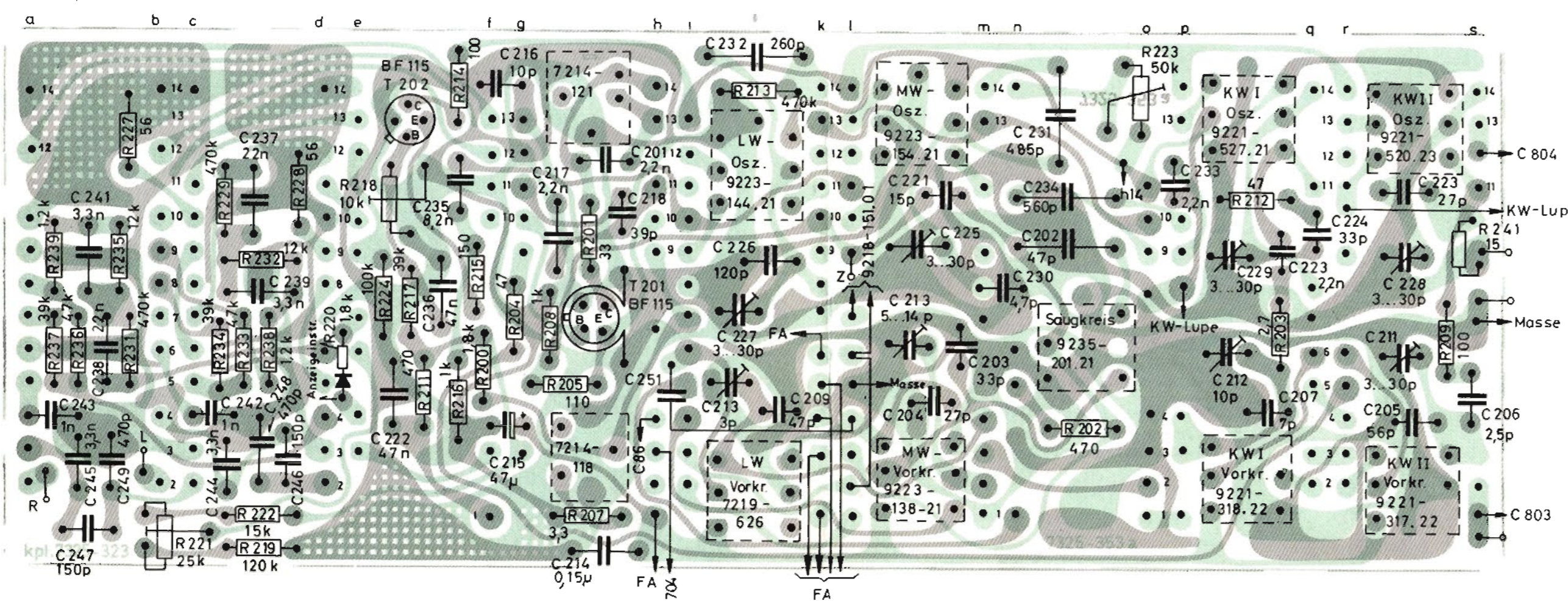
56 V-Platte, Lötseite 56 V PRINTED BOARD, SOLDER SIDE PLAQUETTE 56 V, VUE DU COTE DES SOUDURES PIASTRA 56 V, LATO SALDATURE
