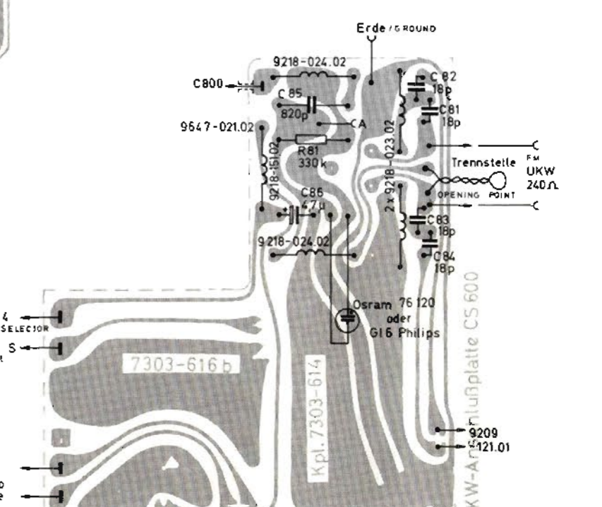
UKW-Anschlußplatte CS 600
