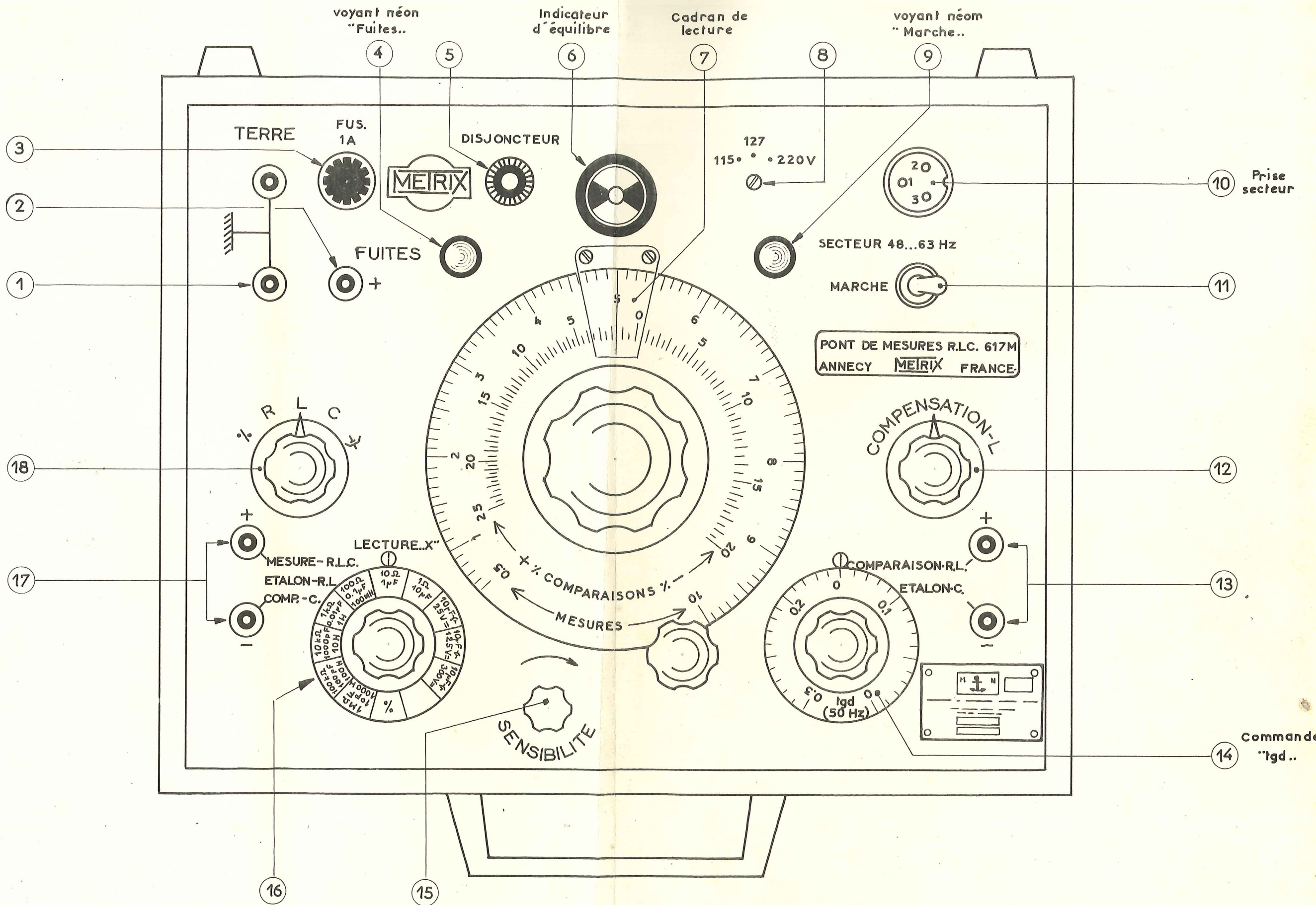
PONT DE MESURES R L C 617M.METRIX VUE AVANT DE L' APPAREIL
