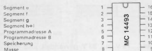
Bild 9 Anschluß-Belegung des MC 14493 IC 205
