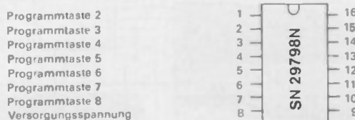
Bild 8 Anschluß-Belegung des SN 29798 IC 208
