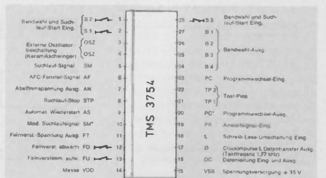
Bild 14 Pin-Belegung TMS 3754
