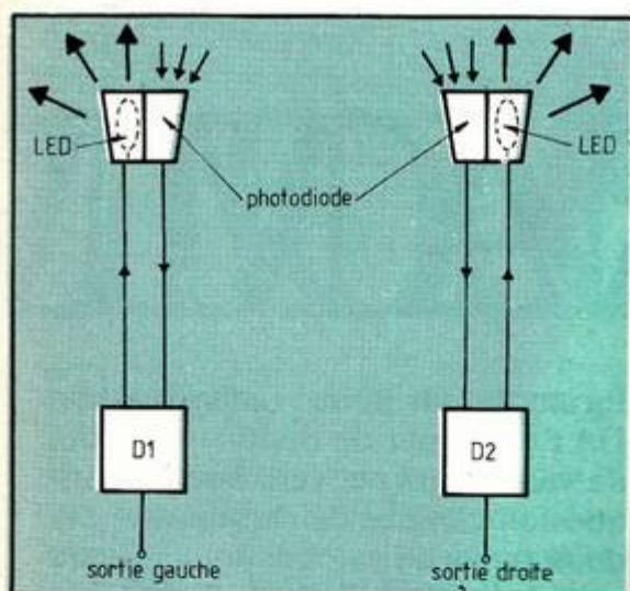
Fig. 16. Disposition des détecteurs.
