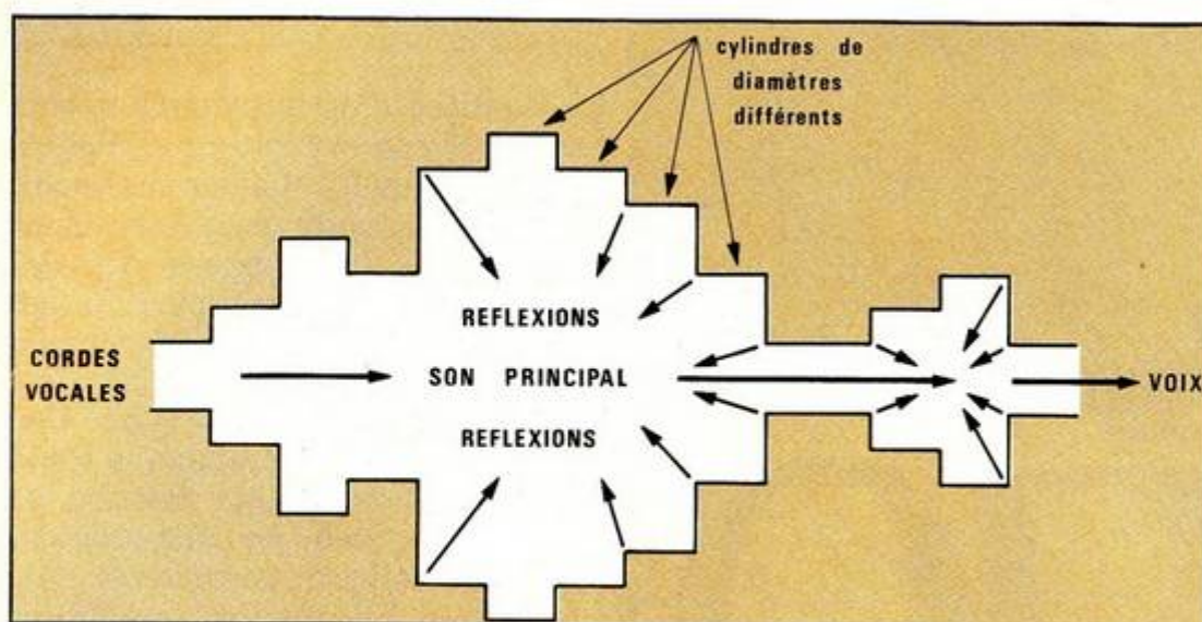
Fig. 3. Modélisation cylindrique du conduit vocal.
