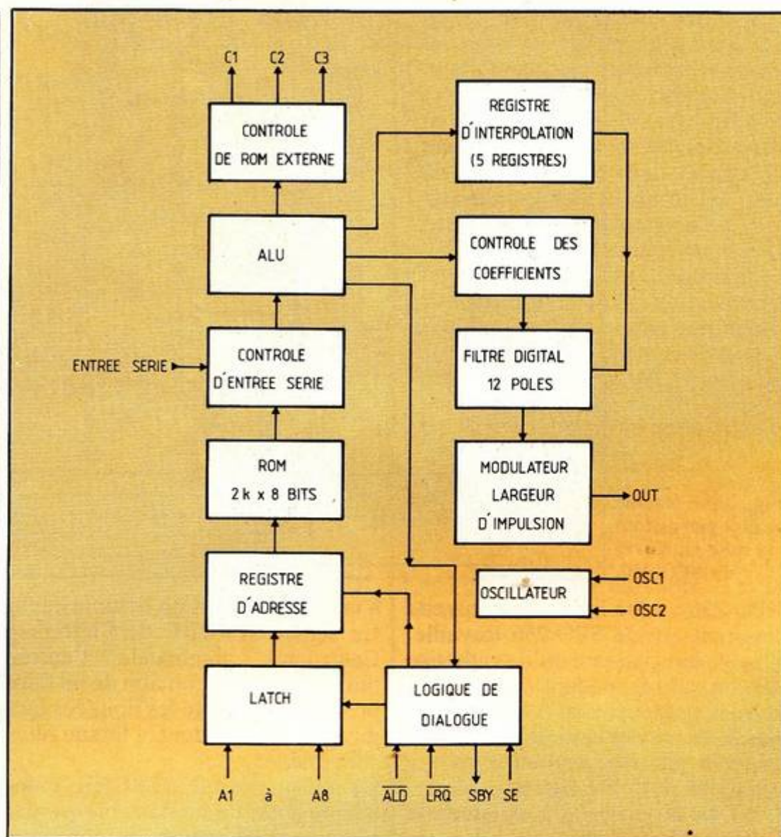
Fig. 1 Synoptique interne du SPO 256.
