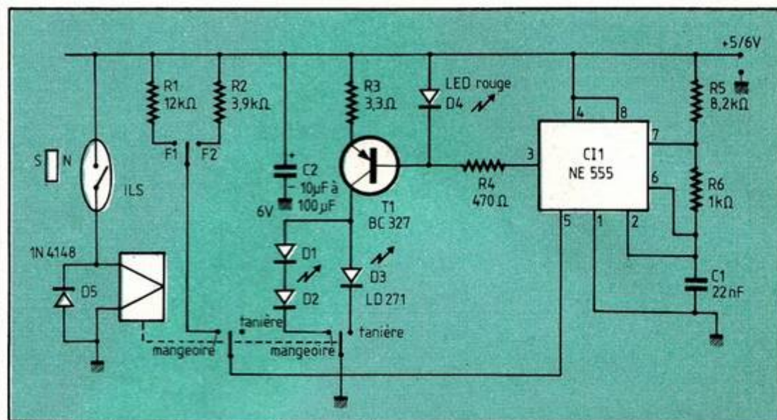
Fig. 1. L'électronique associée aux balises.
