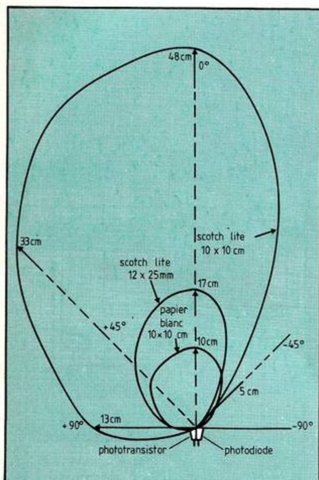
Fig. 14. Diagramme de directivité approximatif du capteur à réflexion.
