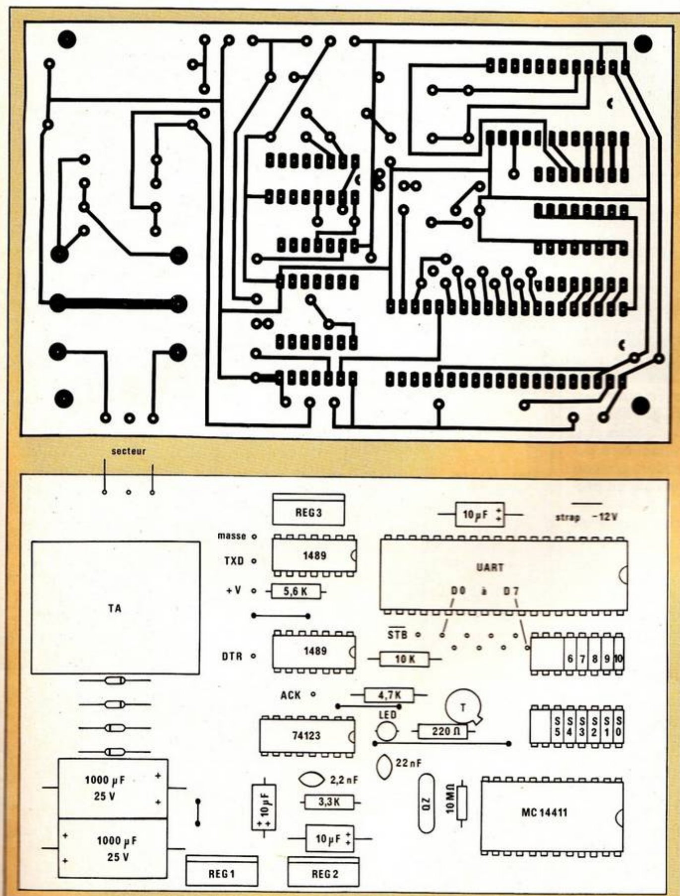
Fig. 5 : Implantation des composants.
