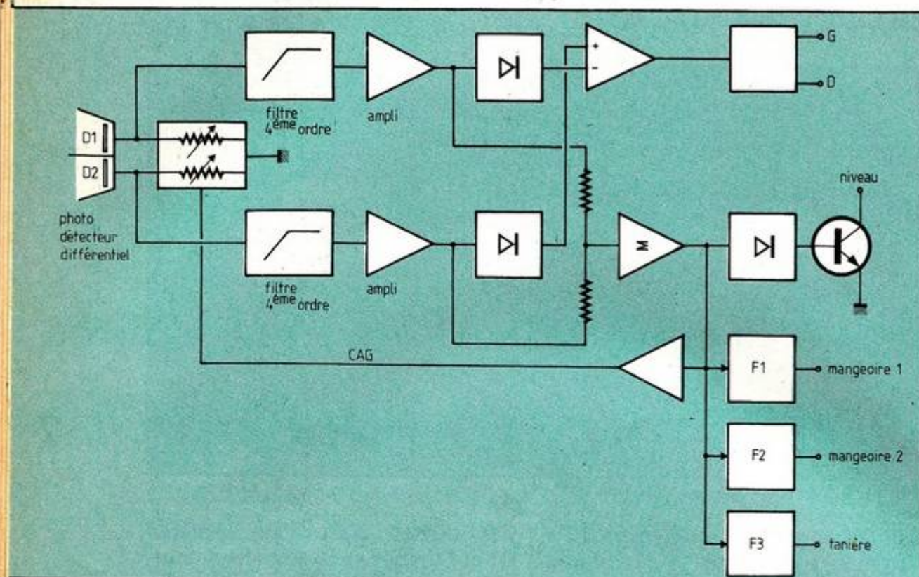
Fig. 2. Synoptique du détecteur directionnel.
