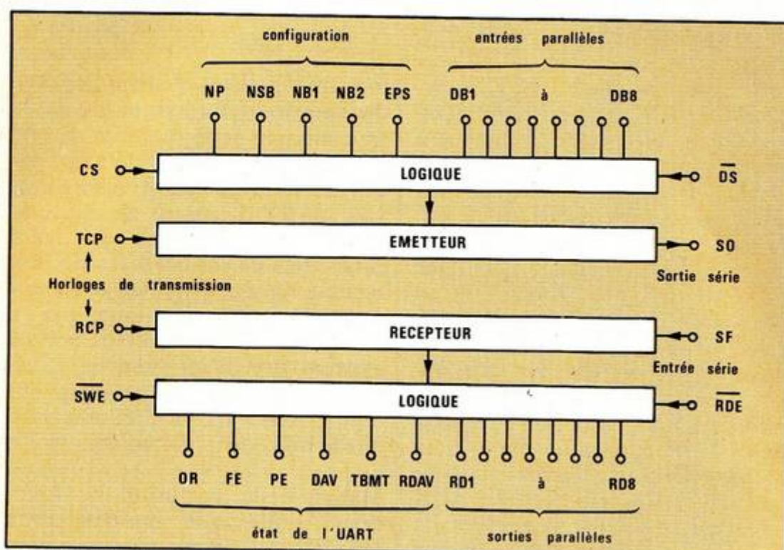
Fig. 2 : Synoptique d'un UART.
