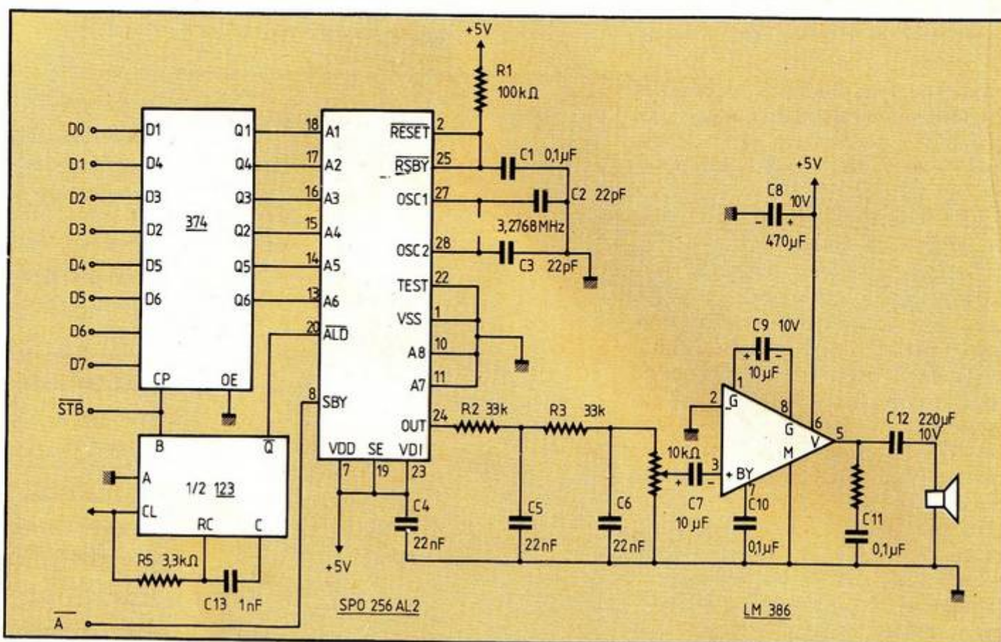
Fig. 2. Le schéma utilisé permettant la mise en œuvre du SPO 256.
