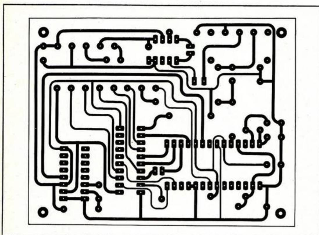
Fig. 4. Circuit imprimé, vu côté cuivre (échelle 1).
