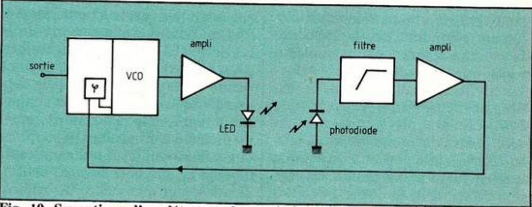
Fig. 10. Synoptique d'un détecteur de proximité.
