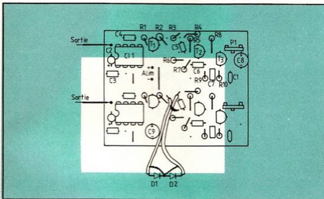
Fig. 13. C.I. du détecteur (éch. 1).
