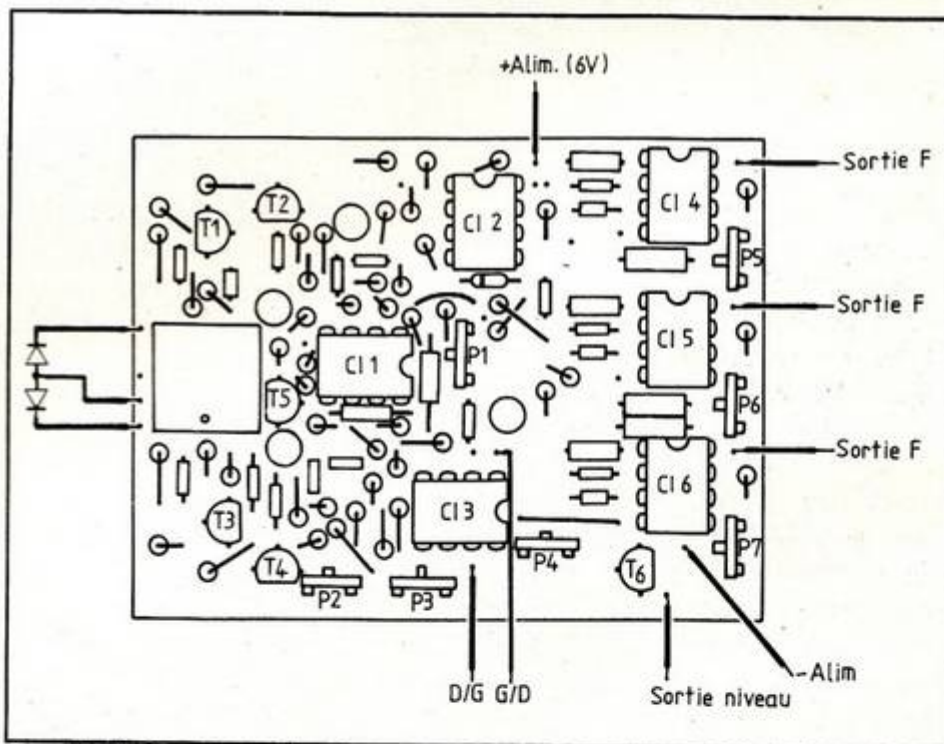
Fig. 7 bis. Implantation des composants du système directionnel.
