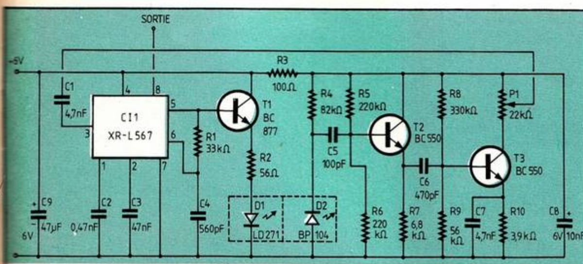
Fig. 11. Schéma du détecteur de proximité opto-électronique.
