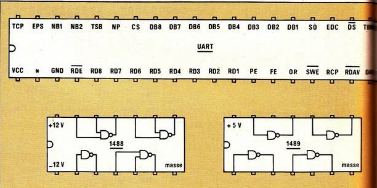
Brochages de l'UART, du 1488 et du 1489.
