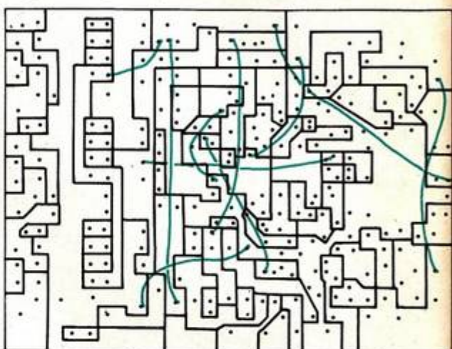
Fig. 8. Câblage des straps (côté cuivre).
