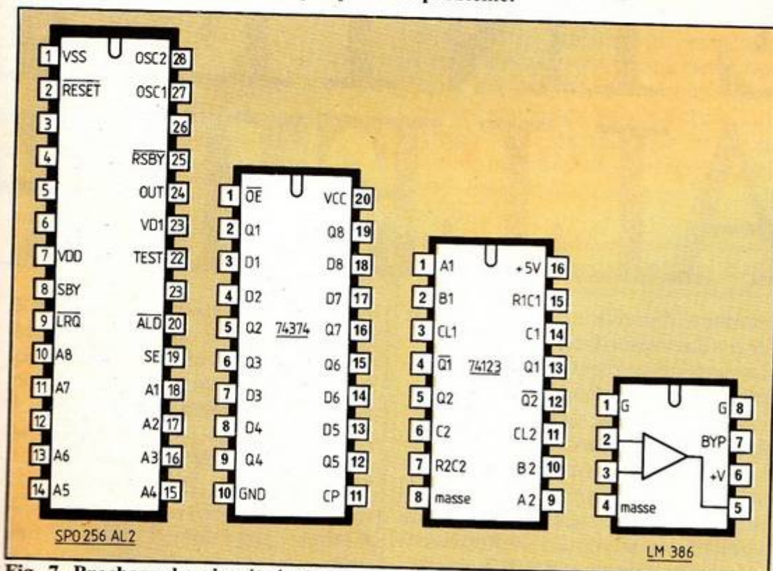
Fig. 7. Brochage des circuits intégrés.
