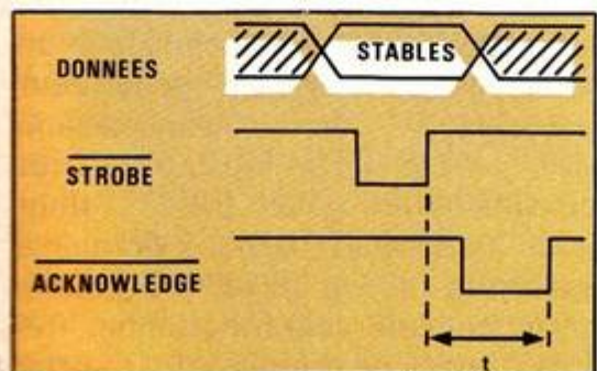
Fig. 1 : Chronogrammes d'une interface Centronics.
