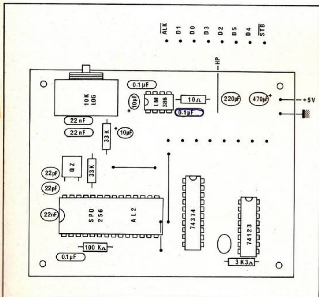
Fig. 5. Implantation des composants.
