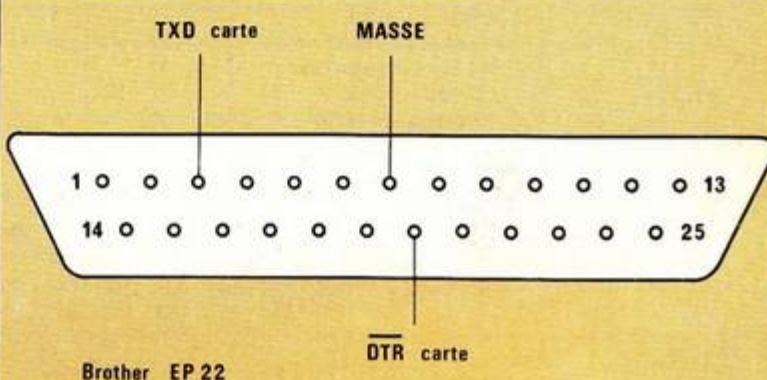
Fig. 6 : Brochages RS 232 et Centronics.
