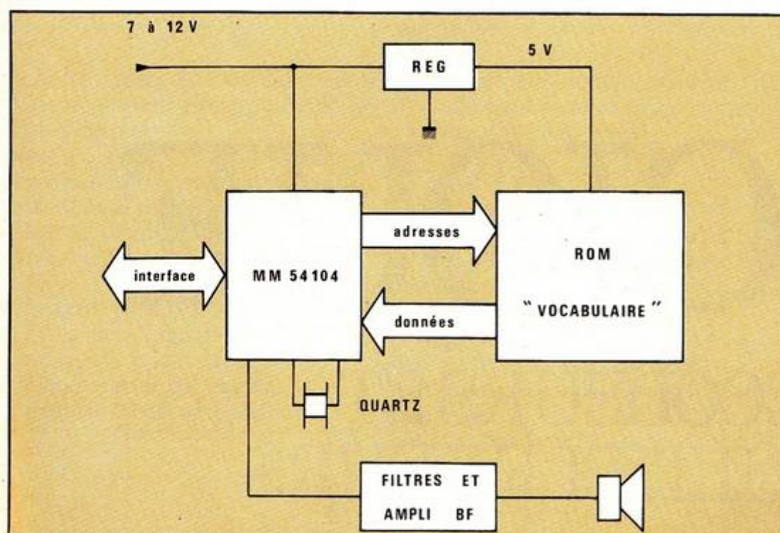
Fig. 4. Exemple de mise en œuvre du processeur N.S.
