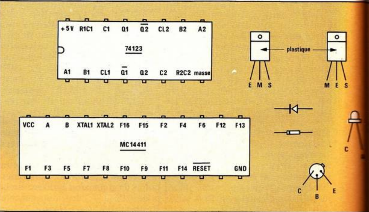
Brochages du 74123, du MC 14411 et des semi-conducteurs.
