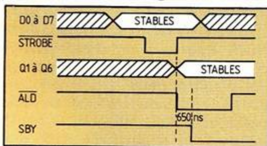
Fig. 3. Chronogrammes de l'interface.
