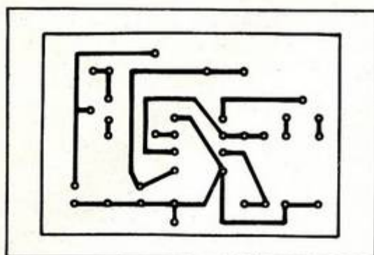
Fig. 4. C.I. de l'émetteur (éch. 1).
