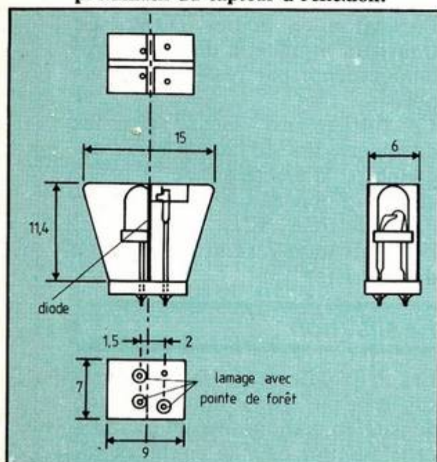
Fig. 15. L'un des capteurs de direction.
