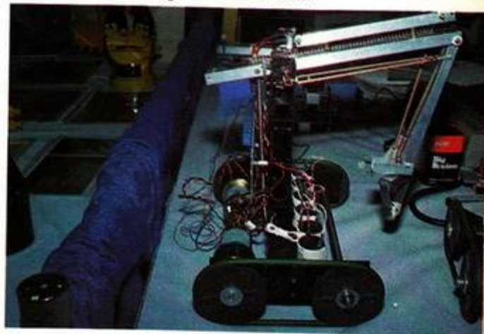
Robot mobile 4 axes de S.I.
