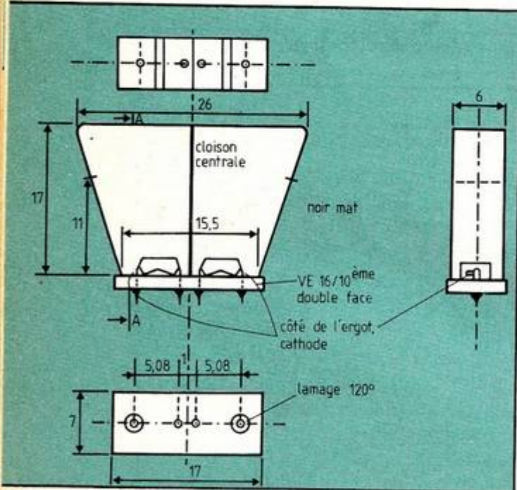
Fig. 9. Plan du capteur de direction. associée à une résistance limitatrice de 470 Ohms. On émet sur la fréquence désirée et on règle le potentiomètre pour que la diode de contrôle s'allume. On repère deux positions d'allumage de part et d'autre et on laisse le potentiomètre au centre, entre les deux positions correspondant à l'allumage. Notez que la position centrale ne correspond pas obligatoirement à la fréquence d'émission : un décalage, normal, peut exister. Le tableau 2 donne les états des sorties en fonction des signaux d'entrée. Il va de soi que le code des sorties de l'indicateur de direction dépend du sens de montage du capteur.
