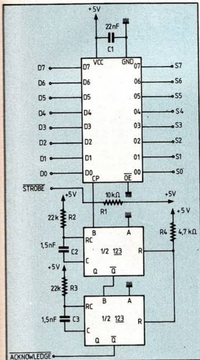
Fig. 3 : le schéma retenu.
