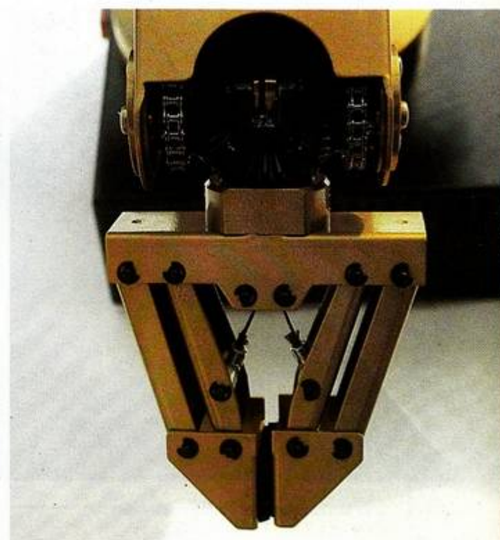
Une pince à deux mors.
