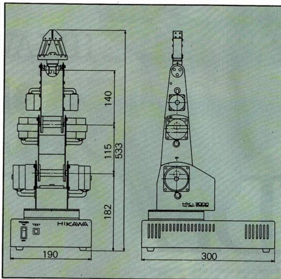
Fig. 1. Les cotes du bras Hikawa HX 3000.
