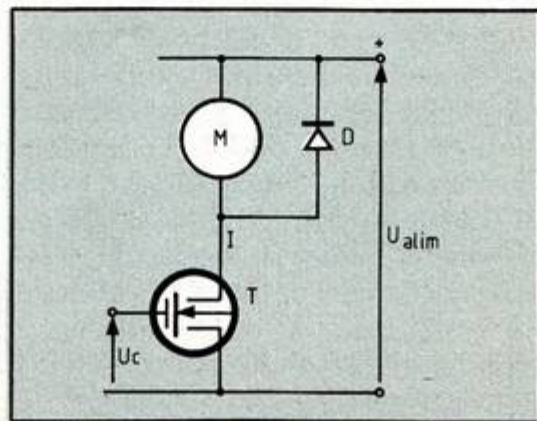
Fig. 3. Commande par Fet de puissance.
