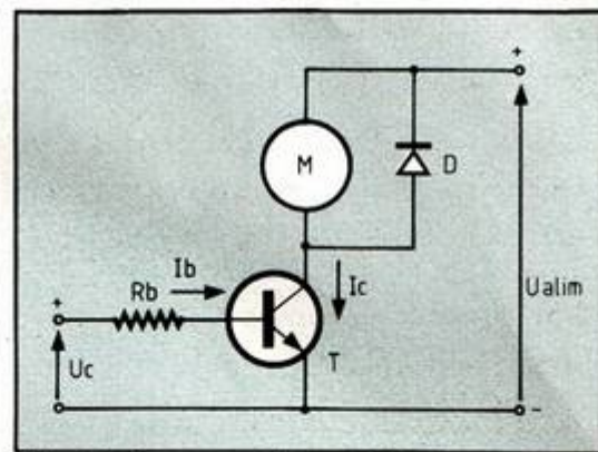
Fig. 1. Commande par NPN.
