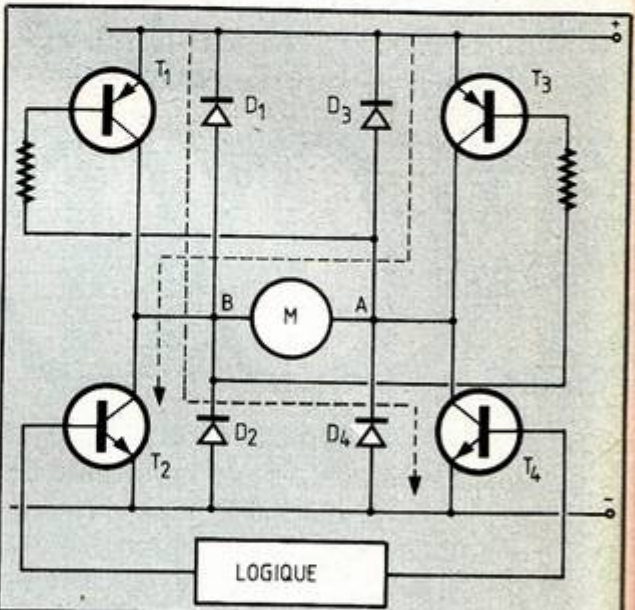
Fig. 7. Montage en pont.
