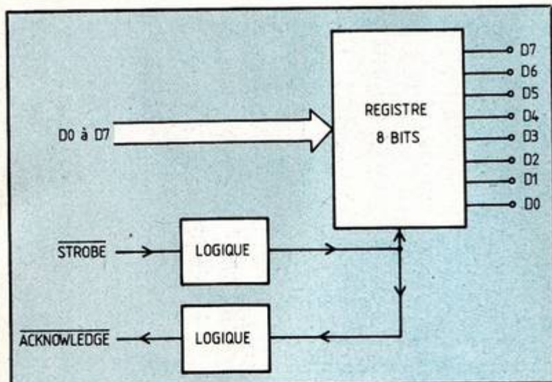
Fig. 2 : le synoptique de cette interface.
