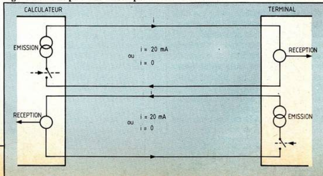
Figure 1 : Principe d'une liaison par boucle de courant.
