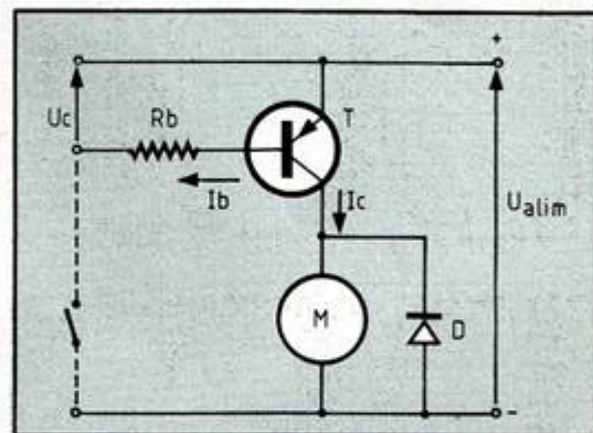
Fig. 2. Commande par PNP.
