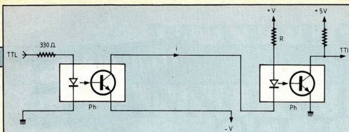
Figure 2 : Boucle de courant réalisée par photo-coupleurs.
