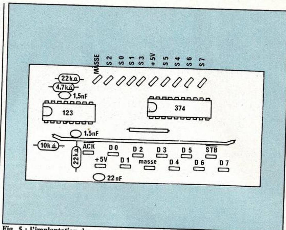
Fig. 5 : l'implantation des composants.
