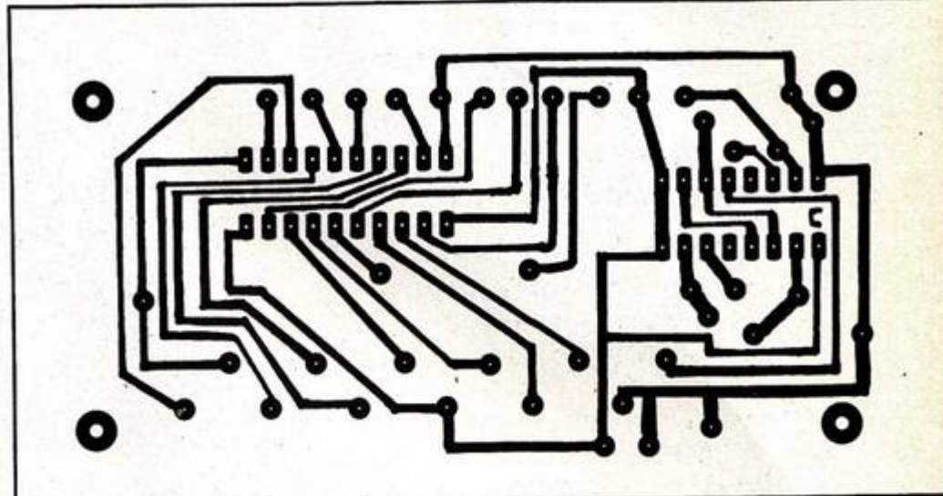
Fig. 4 : le circuit imprimé, côté cuivre (éch. 1).
