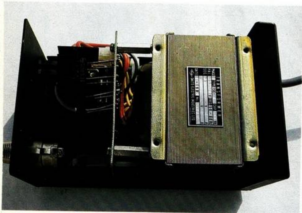
L'intérieur de l'alimentation.
