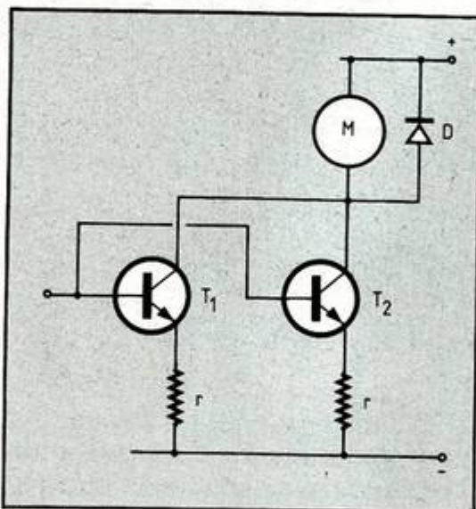
Fig. 4. Commande avec NPN en parallèle.
