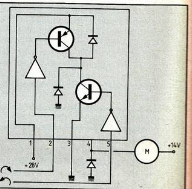
Fig. 8. L'UDN 2949Z de Sprague.
