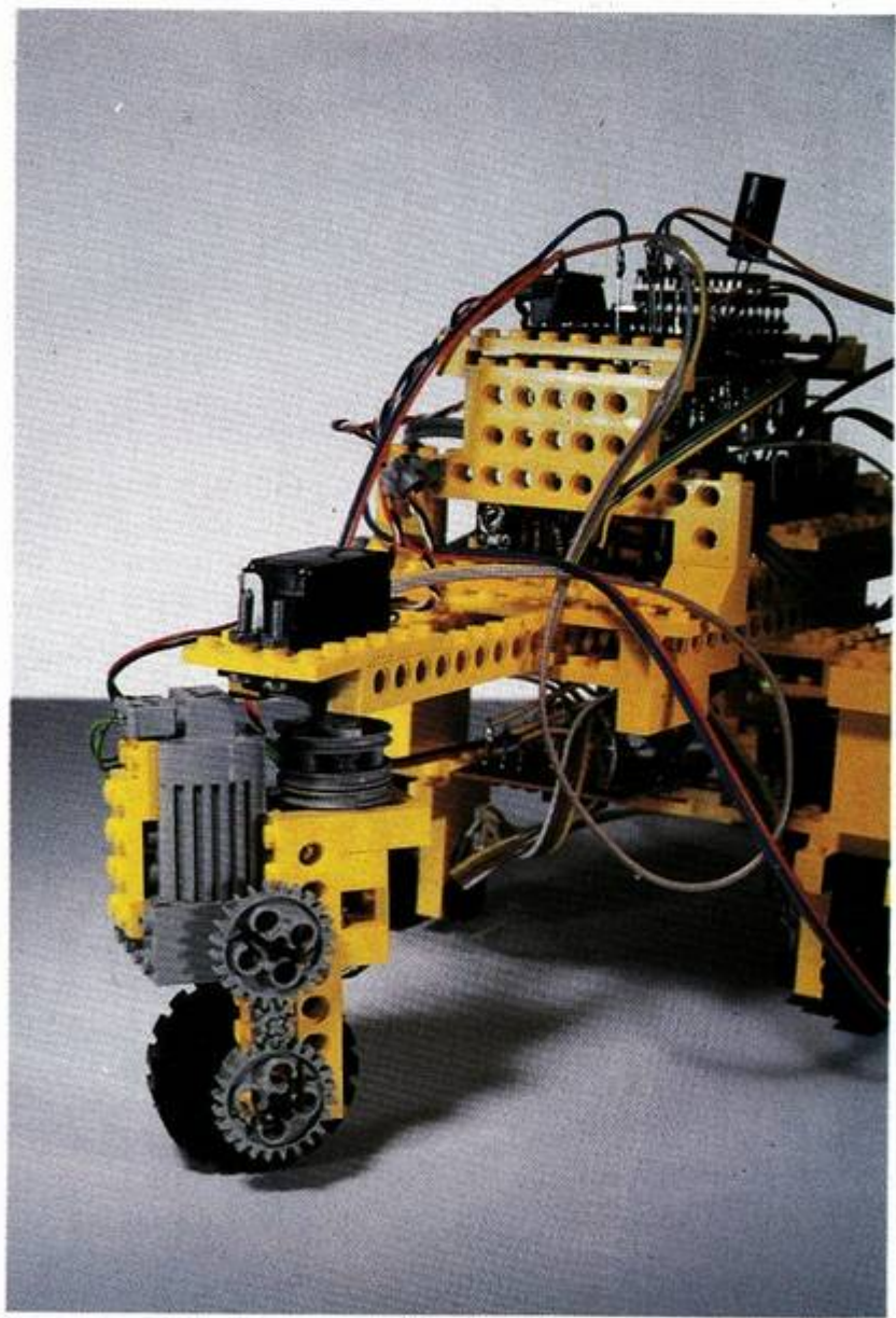
La roue motrice assure aussi la direction.
