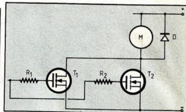
Fig. 5. Fet mis en parallèle.
