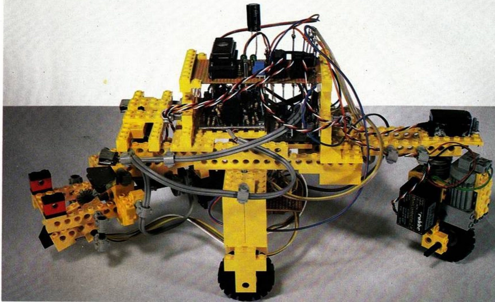
Le Cybernoid dans sa phase expérimentale et sous sa forme quasi définitive.
