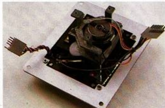
La platine mécanique du Memocom.
