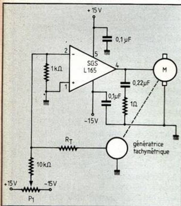
Fig. 9. Commande par CI de puissance.
