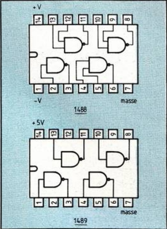
Figure 6 : Brochages des 1488 et 1489.
