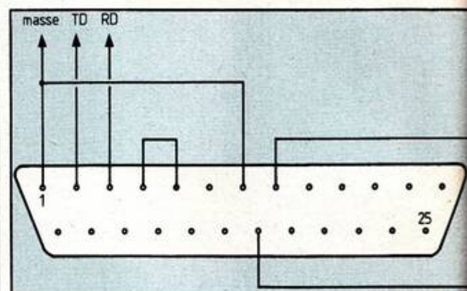
Fig. 8 : Bouchon de court-circuit pour liaison RS232 incomplète.
