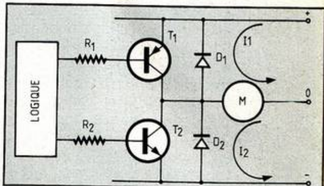
Fig. 6. Montage en demi-pont.
