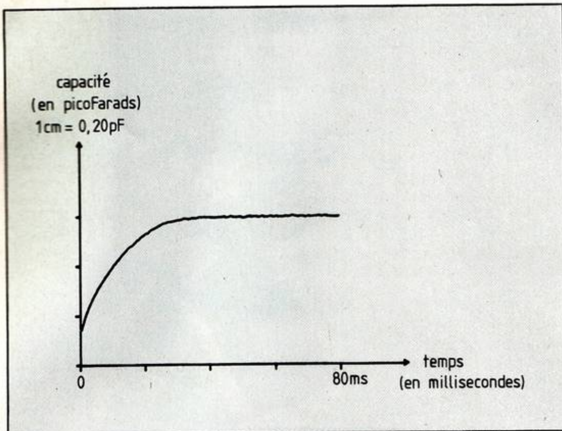
Fig. 2. Transitoire de capacité : le dépouillement par la méthode «DLTS» (Deep Level Transient Spectroscopy) donne une seule composante, avec un décrement T = 35 ms. Le signal est donc analysé comme C(t) = a - b \exp(-t/T) + \text{bruit} . Une analyse par la méthode suggérée du § 1.4 donnerait-elle des résultats différents ? (Documentation : Groupe de physique des solides, Paris 6).
