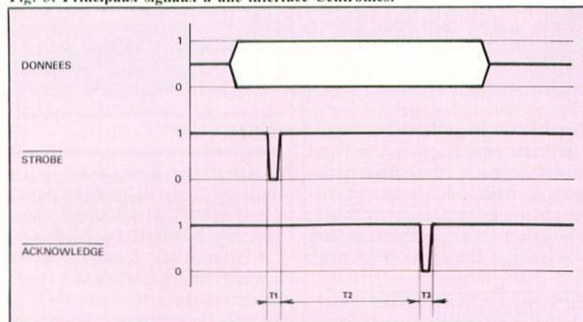
Fig. 3. Principaux signaux d'une interface Centronics.
