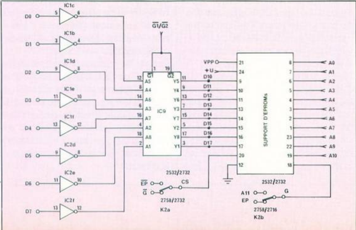
Fig. 5. Schéma de principe de l'interface. Les broches D10 à D17 constituent le bus des données.
