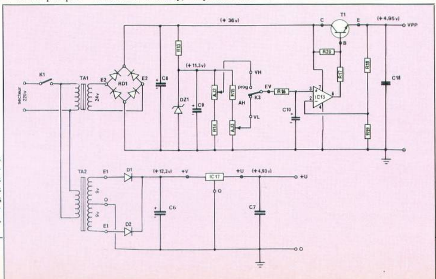
Fig. 9. Les alimentations + 25 V et + 5 V. Les valeurs indiquées entre parenthèses ont été relevées sur la maquette.
