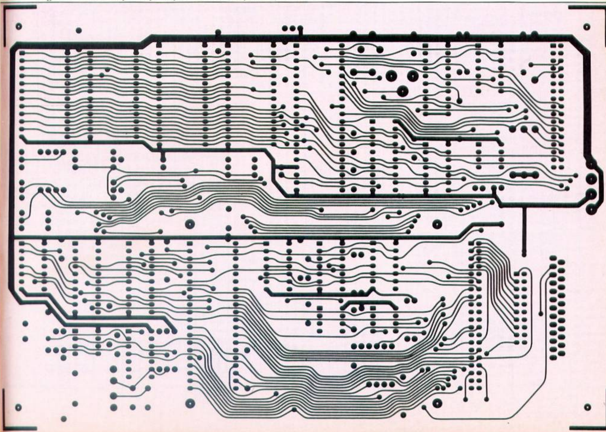
Figure 3. Circuit imprimé principal, vu côté composants, échelle 1.
