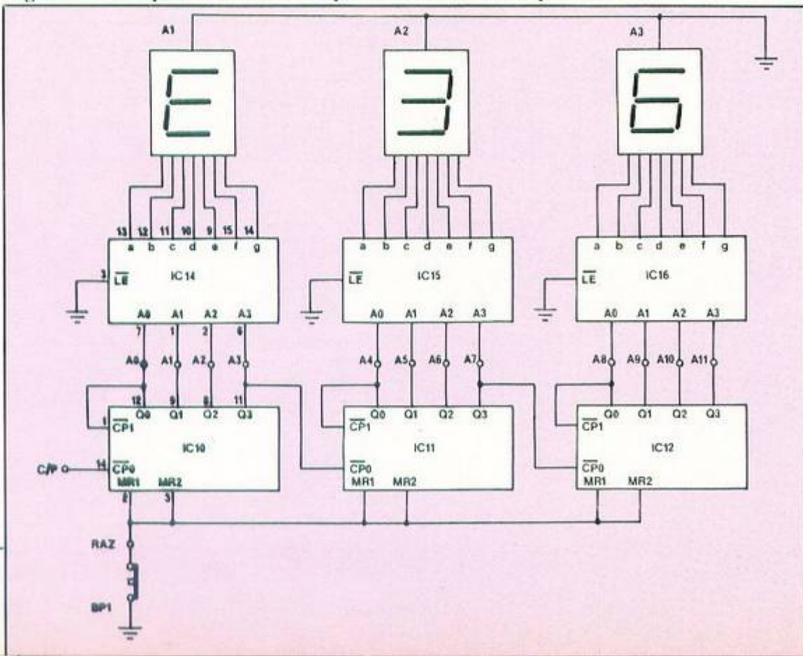
Fig. 8. Le compteur est réalisé à partir de 3 diviseurs par 16.
