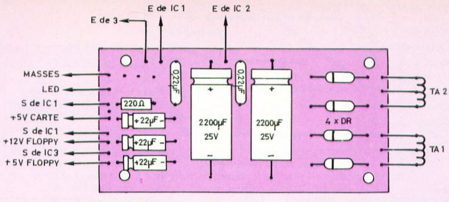
Figure 5. Implantation des composants sur le circuit imprimé de l'alimentation.
