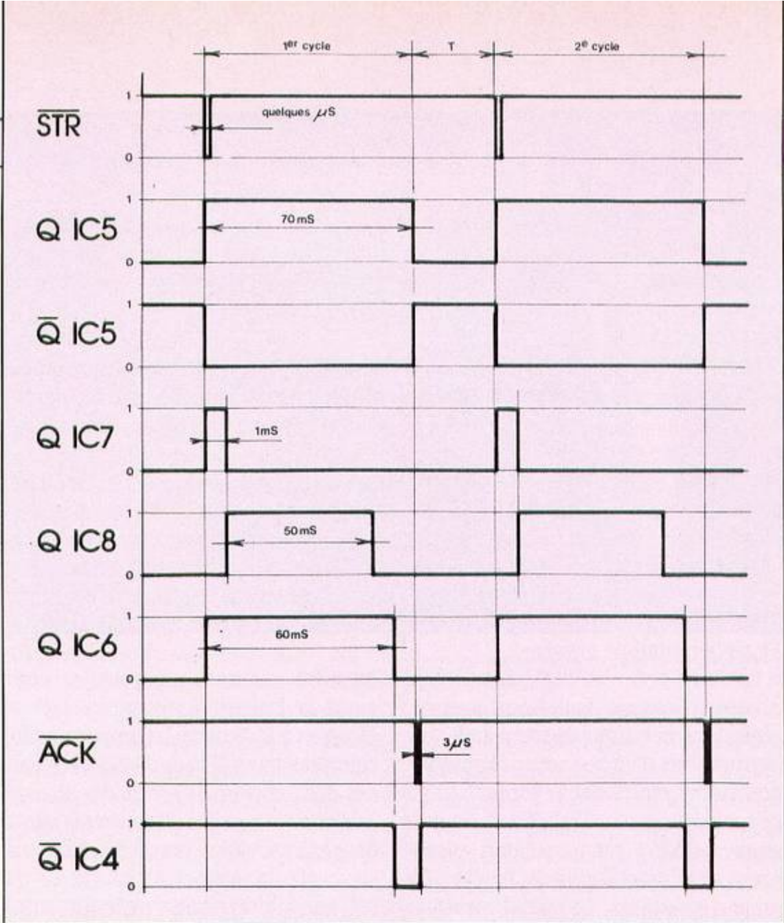
Fig. 7. Chronogramme des principaux signaux délivrés par la logique de commande. la rapidité du logiciel lequel, s'il est écrit en BASIC, peut allonger cette durée dans des proportions non négligeables.
