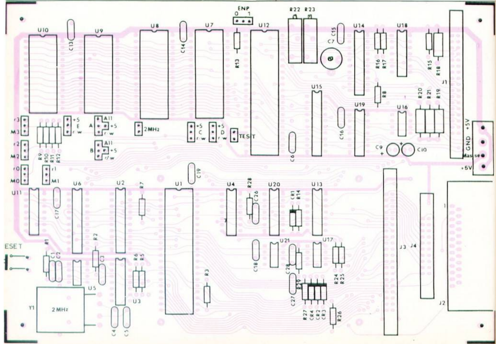
Figure 6. Implantation des composants sur le circuit imprimé principal.
