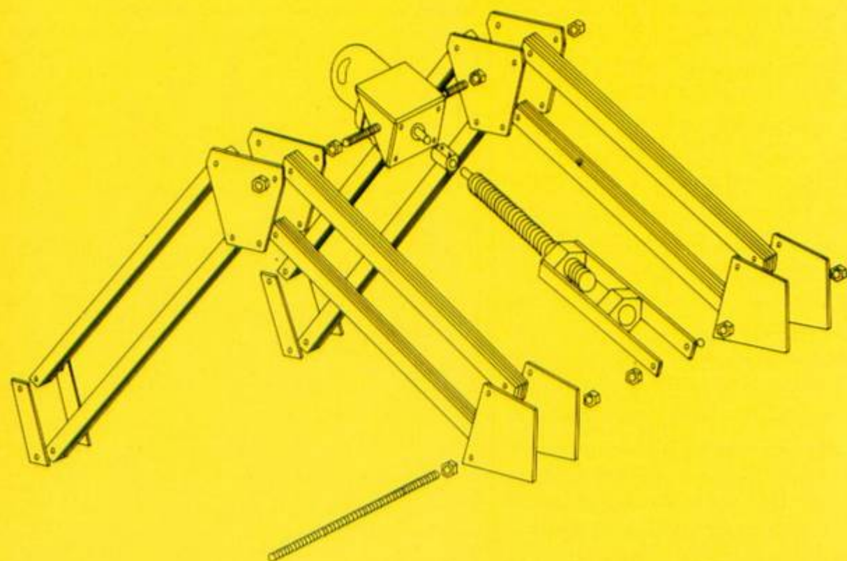
Figure 7 : l'assemblage des pièces constituant le bras.
