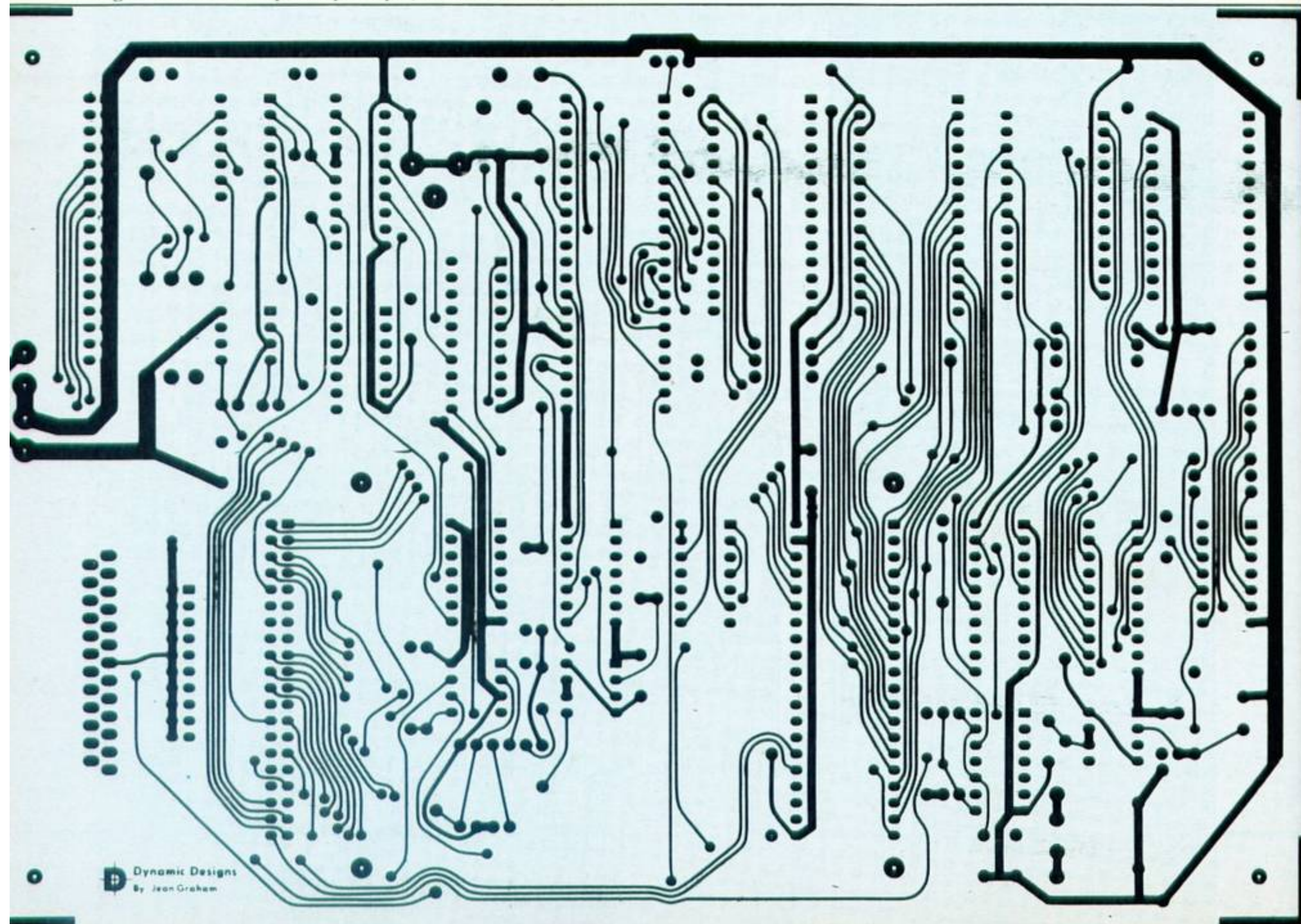
Figure 2. Circuit imprimé principal, vu côté cuivre, échelle 1.
