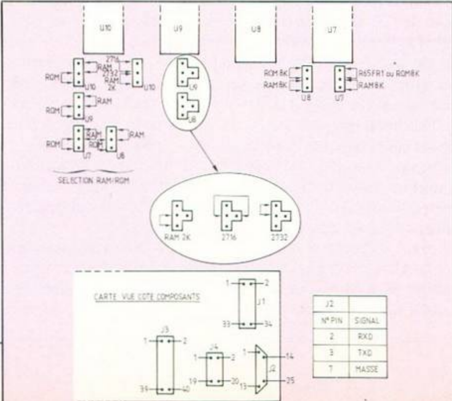
Figure 8. Positionnement des straps de sélection des types de mémoires.
