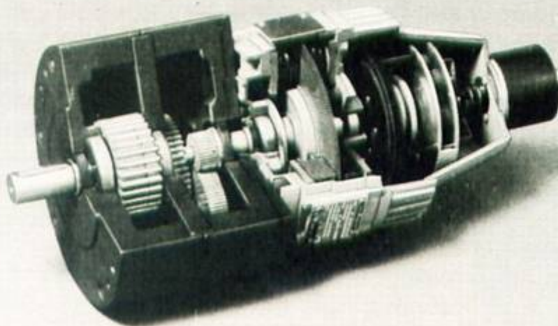
Exemple d'adaptation Axem MC + tachy + codeur + frein + réducteur
