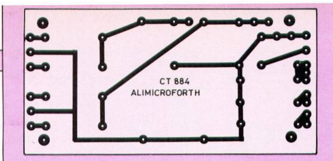
Figure 4. Circuit imprimé de l'alimentation, vu côté cuivre, échelle 1.
