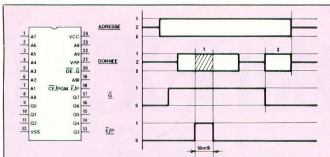
Fig. 1. Brochage et programmation des 2758 et 2716. Phase 1 : programmation ; phase 2 : restitution de la donnée.
