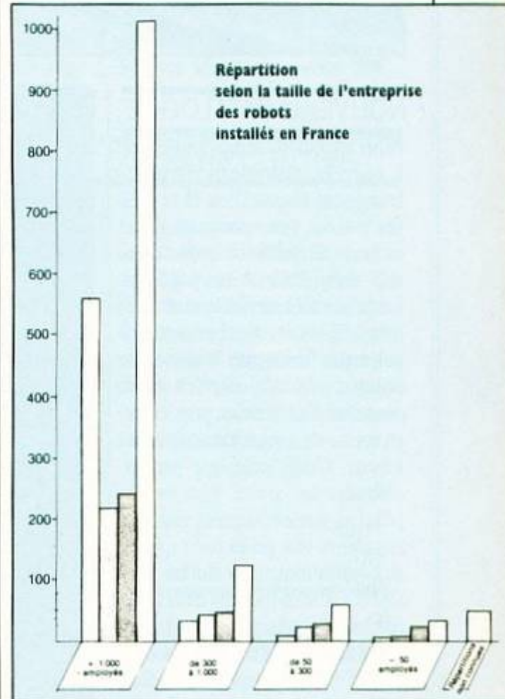
Répartition des robots installés en France, selon la taille de l'entreprise. 1 re colonne : robots d'origine française ; 2 e : robots d'origine européenne moins la France ; 3 e : robots d'origine mondiale moins l'Europe ; 4 e : total des robots. Source : Axes Robotique.
