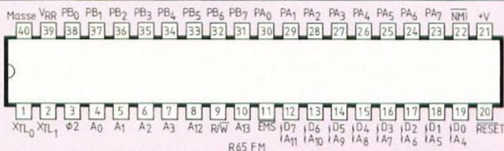
Figure 10. Brochage des circuits intégrés.
