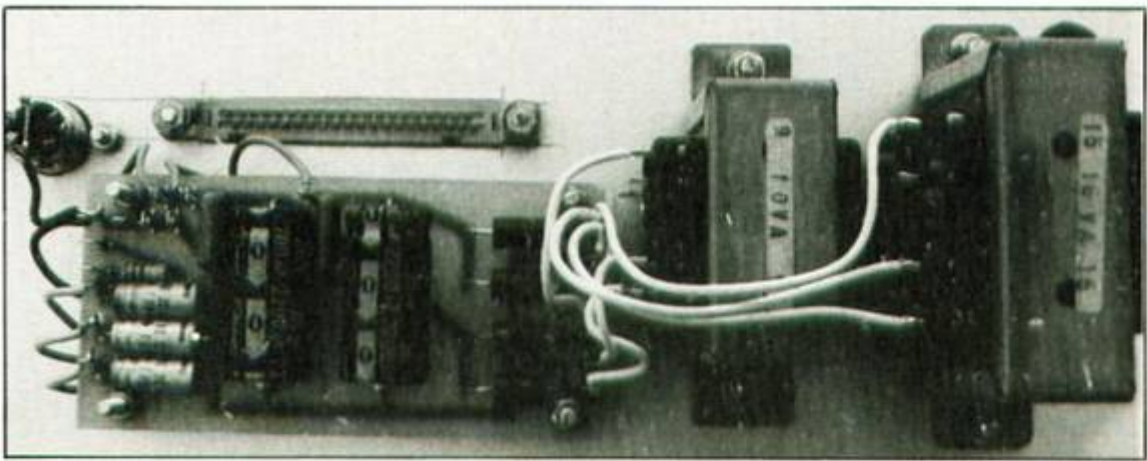
Le circuit imprimé de l'alimentation et les transformateurs.
