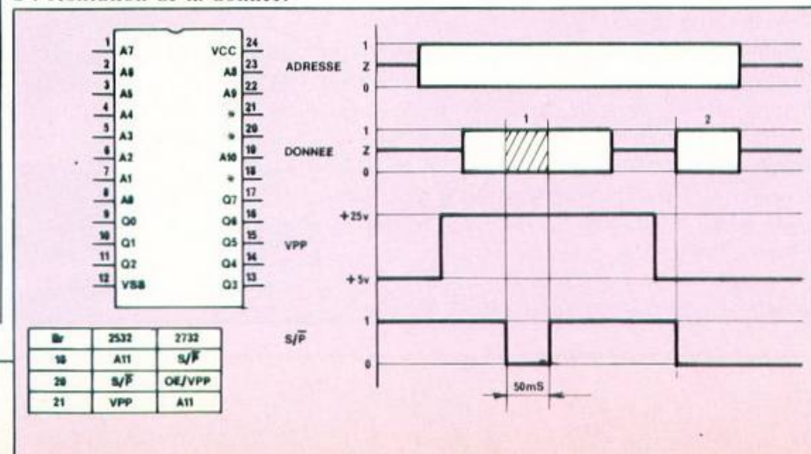
Fig. 2. Brochage et programmation des 2532 et 2732. Phase 1 : programmation ; phase 2 : restitution de la donnée.
