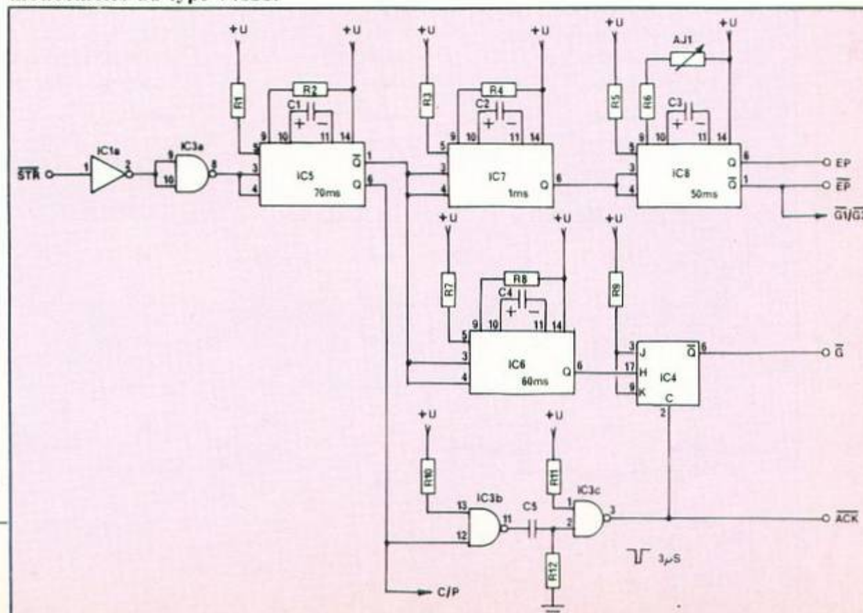
Fig. 6. La logique de commande : la plupart des informations sont fournies par des monostables du type 74121.
