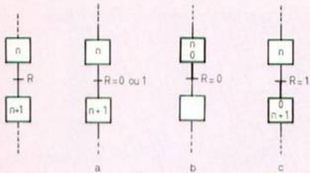
Fig. 5 a) : transition non validée, étape n inactive. b) : transition validée, étape n active mais non franchie, R = 0 . c) : transition franchie car R = 1 alors qu'elle était validée.
