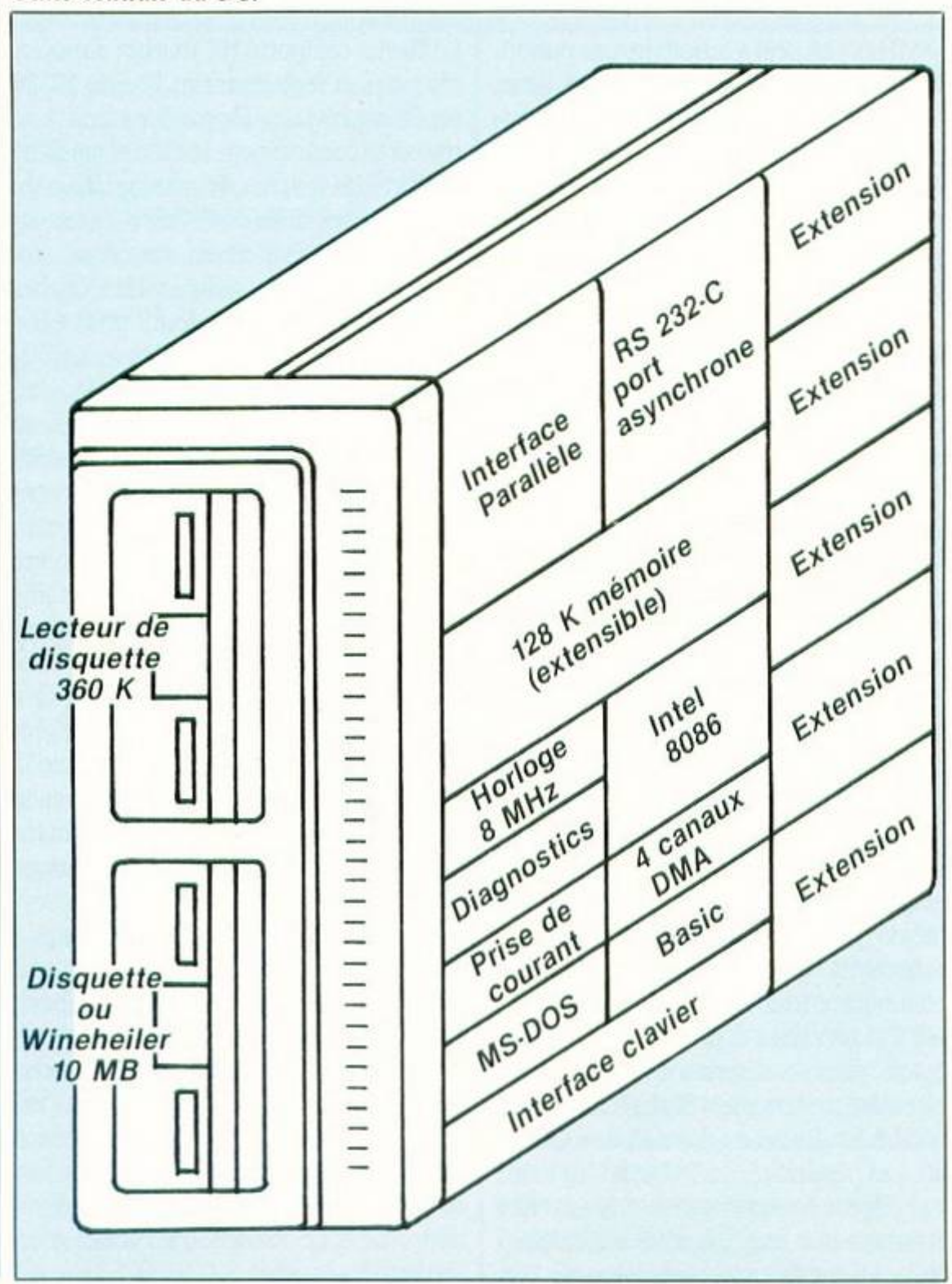
Unité centrale du PC.
