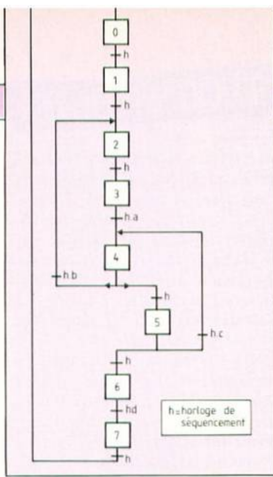
Figure 11a. veau programme dans la mémoire et ce, sans toucher au câblage et en gardant une bonne vitesse d'exécution (contrairement aux systèmes macroprogrammés à base de microprocesseurs). Exemple de séquenceur synchrone Prenons un exemple de système où les 3 évolutions (enchaînements, sauts, arrêts) coexistent. Ce système est décrit soit — par un Grafcet (figure 11a) ; — par un organigramme (figure 11b). Figure 11b.
