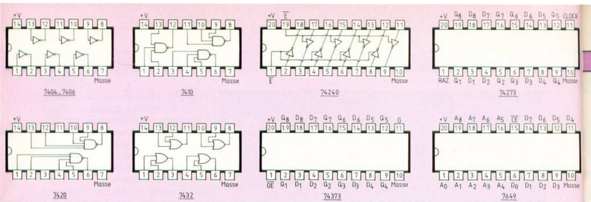
Figure 10. Brochage des circuits intégrés.
