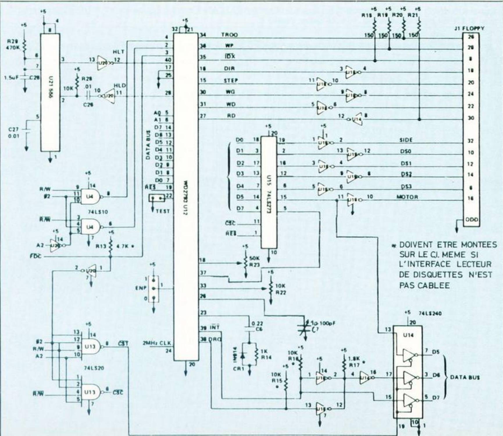
Figure 1. Le sous-ensemble interface lecteurs de disquettes.
