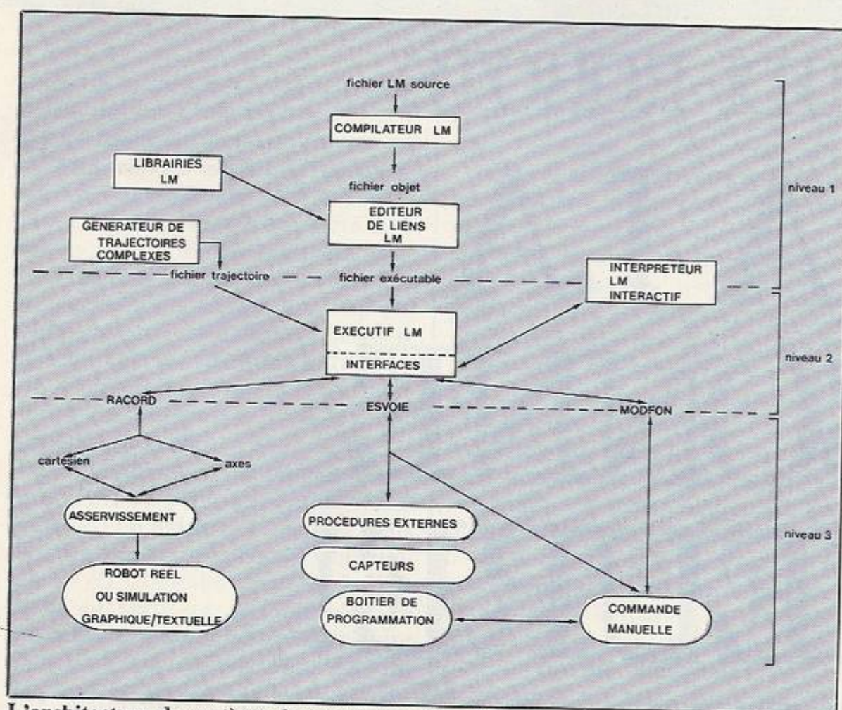
L'architecture du système de programmation LM.
