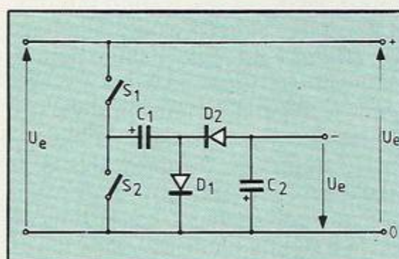
Figure 8. Variante de la figure 7 pour obtenir une tension négative.
