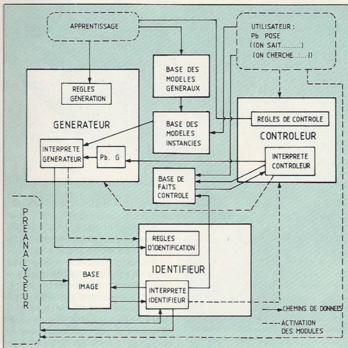
L'architecture de base du système Sacso.
