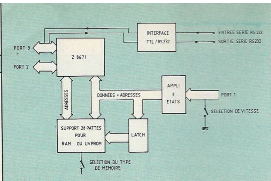
Figure 2. Synoptique de l'automate décrit.
