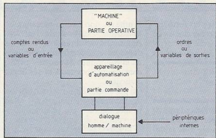
Figure 1a. La partie commande et la partie opérative d'un système automatisé.
