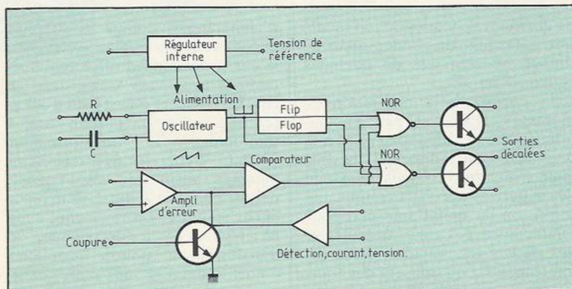
Figure 4. Schéma de principe d'un circuit intégré spécifique aux alimentations à découpage.
