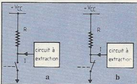
Figure 12. Etat bas (a) ou haut (b) si capteur actionné.
