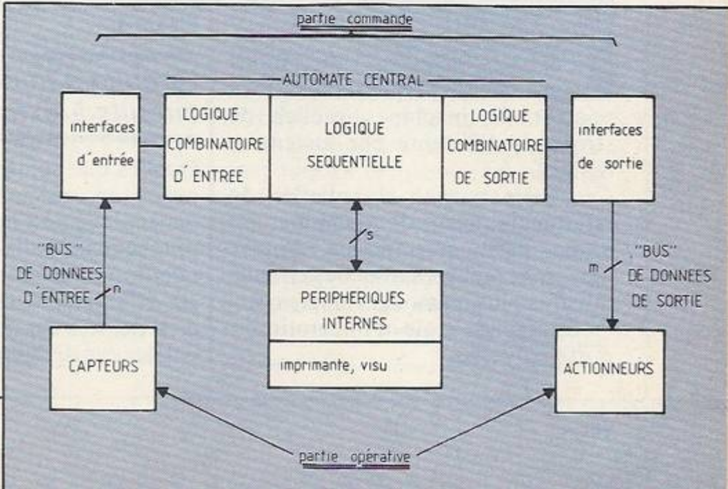
Figure 1b. Le synoptique d'un automate industriel.
