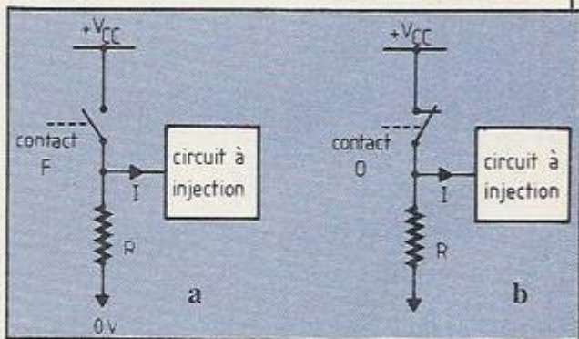
Figure 11. Etat haut (a) ou bas (b) si capteur actionné.
