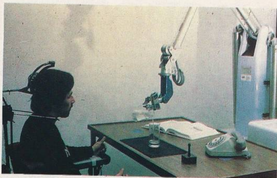
Spartacus : l'aide aux tétraplégiques.
