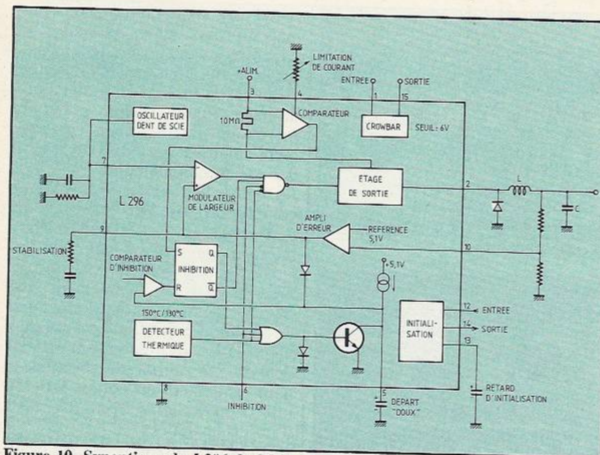
Figure 10. Synoptique du L296 de SGS.
