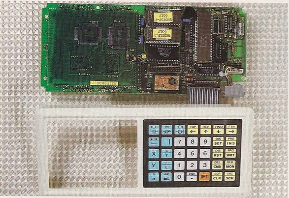
L'intérieur du boîtier de commande de l'AOIP.
