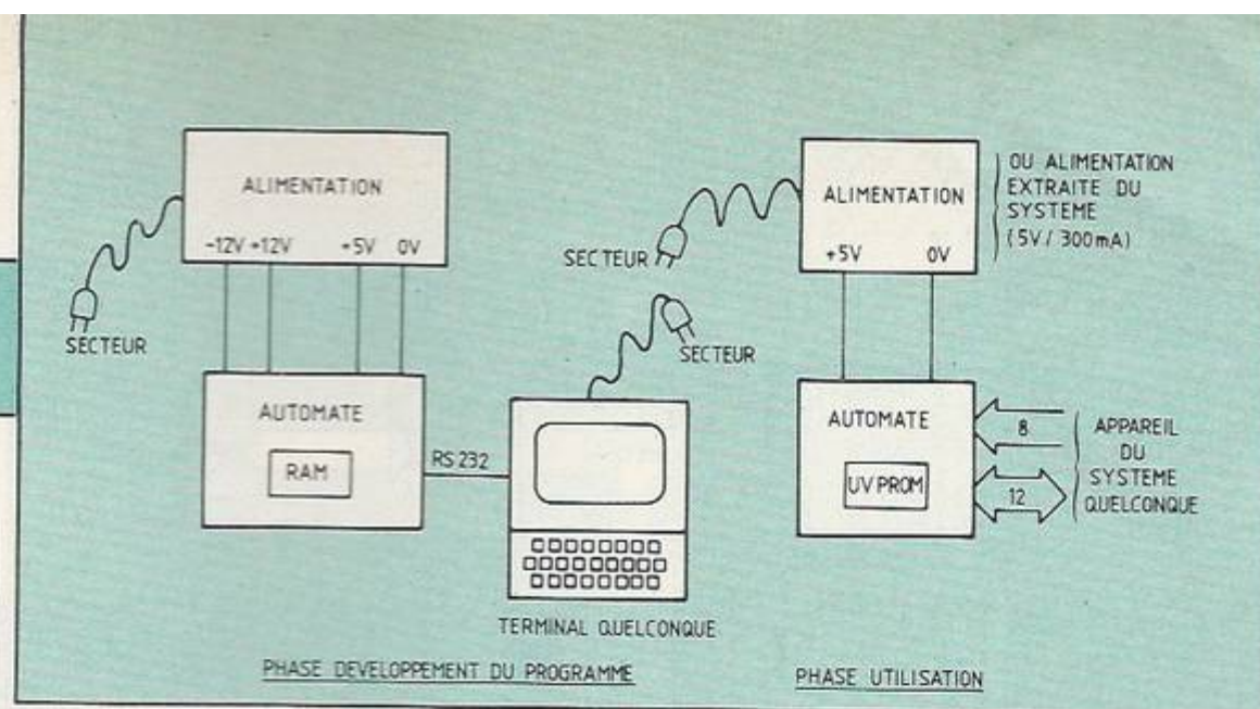
Fig. 1 Les deux modes de fonctionnement de la carte.
