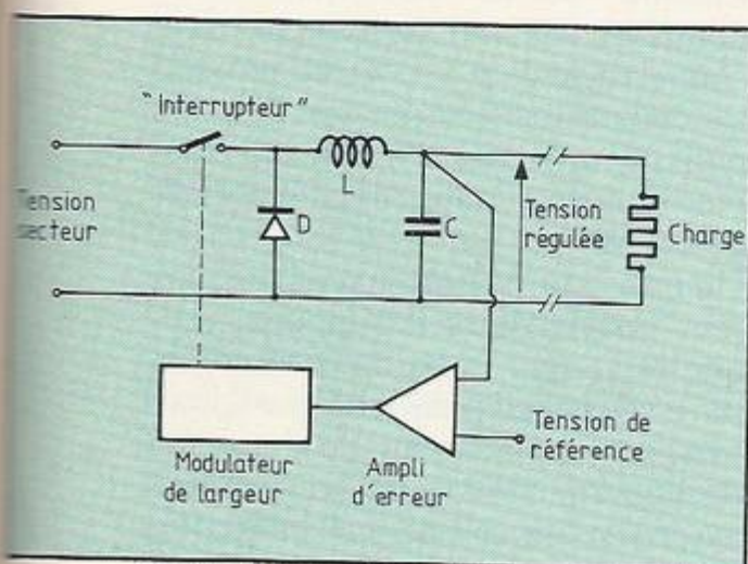
Figure 2. Principe de l'alimentation à découpage régulée.
