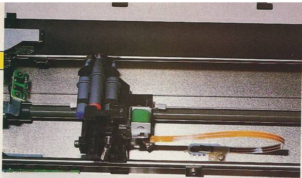
La tête d'impression montée sur un chariot.
