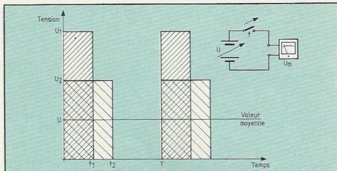
Figure 1. Trois possibilités pour obtenir la même tension moyenne : U_1.t_1 = U_2.t_2 = U.T .
