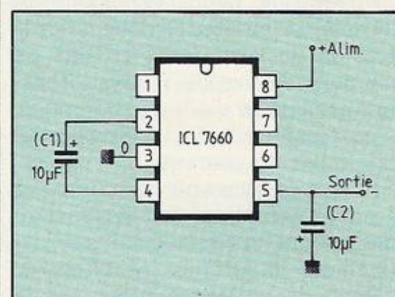
Figure 9. Schéma de principe du montage des CI Intersil.
