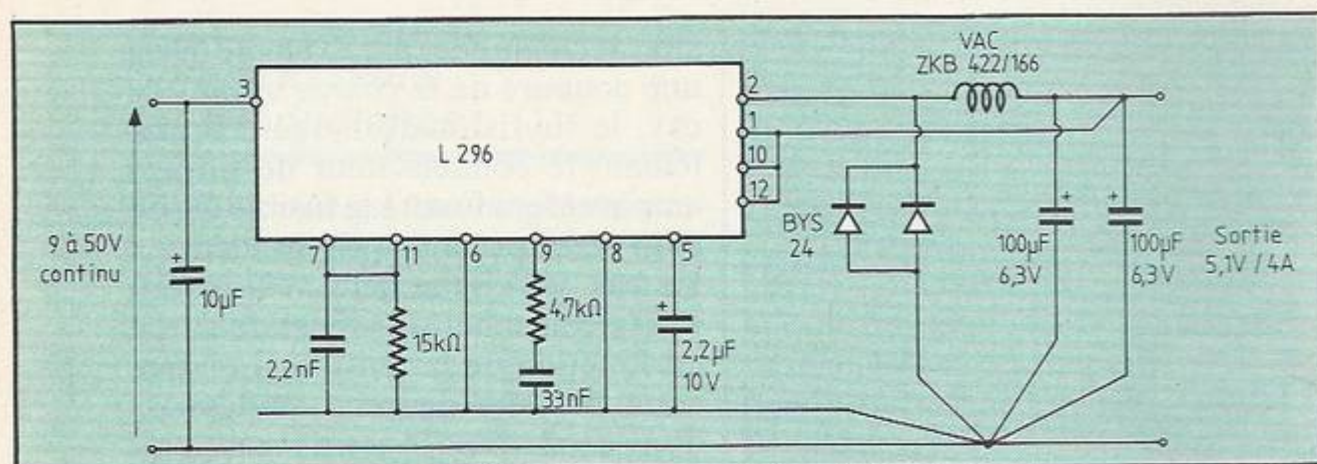
Figure 11. Le schéma minimal retenu pour l'expérimentation.
