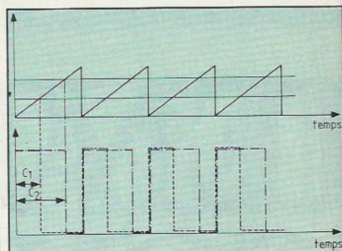
Figure 5. Principe de commande du temps de passage adopté dans la plupart des circuits intégrés.
