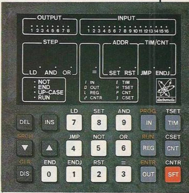
La face avant de l'Electromatic.
