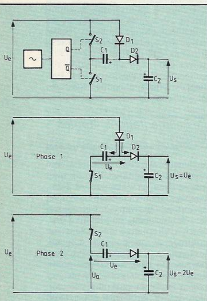
Figure 7. Doublage de tension sans transformateur ni inductance.
