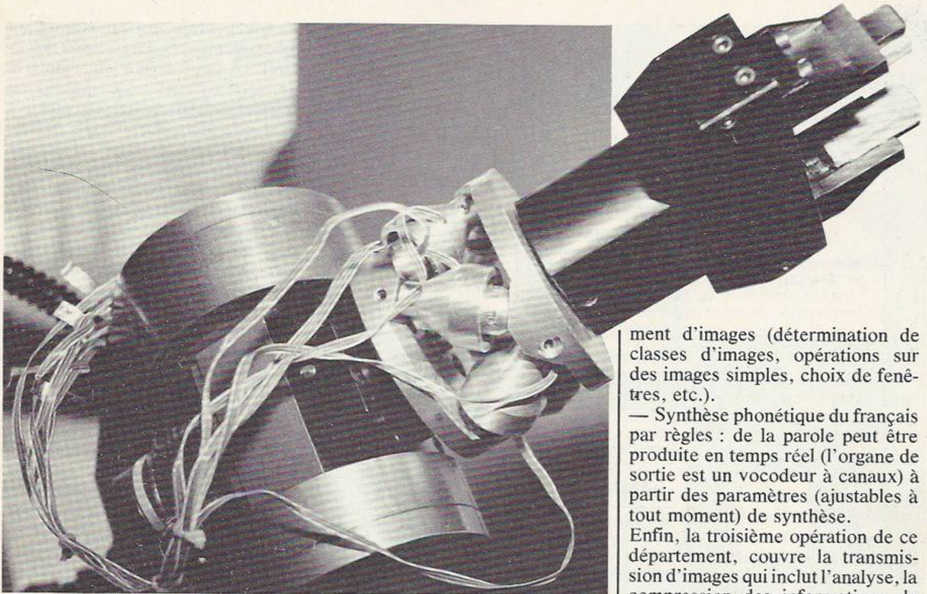
Cert-Onera : une structure en treillis pour ce splendide capteur d'effort 6 axes, ici monté sur l'excellent robot de la société Scemi.
