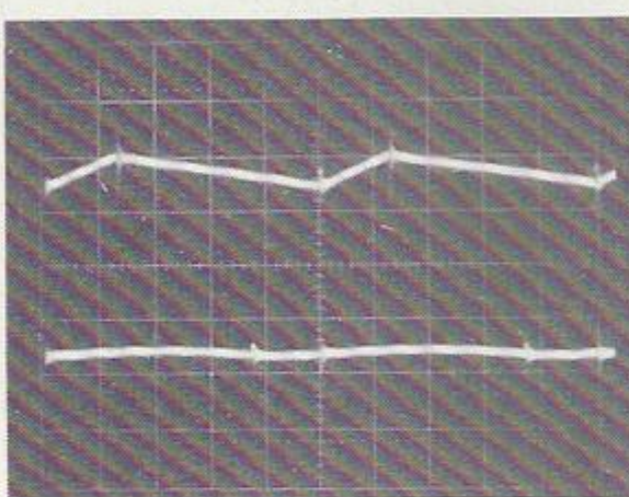
A. Oscillogramme de la tension alternative de sortie superposée à la tension continue de 5 V. En haut, nous avons une seule cellule de filtrage; en bas une seconde, moins efficace (inductance de 20 µH) a été ajoutée. Les signaux transitoires ont, en réalité, une amplitude supérieure, leur faible luminosité ne permet pas de les voir correctement. La sensibilité verticale est de 50 mV/division et l'échelon de temps de 5 µs/division.
