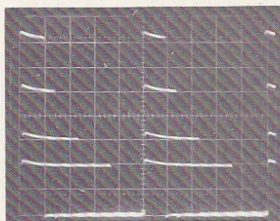
B. Ici, nous avons superposé la tension de sortie du circuit intégré obtenue pour plusieurs valeurs de la tension amont. On notera la variation du temps de passage du courant en fonction de la tension d'alimentation, ce qui justifie la théorie! Echelle verticale : 5 V/division, horizontale : 5 µs/division.
