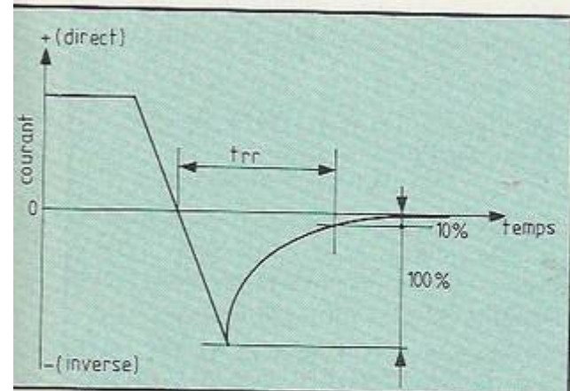
Figure 6. Diagramme permettant de définir le temps de recouvrement d'une diode en commutation.
