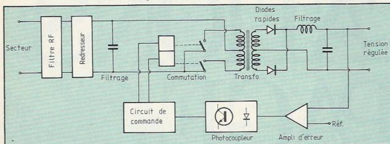
Figure 3. Schéma synoptique d'une alimentation à découpage à partir du secteur.
