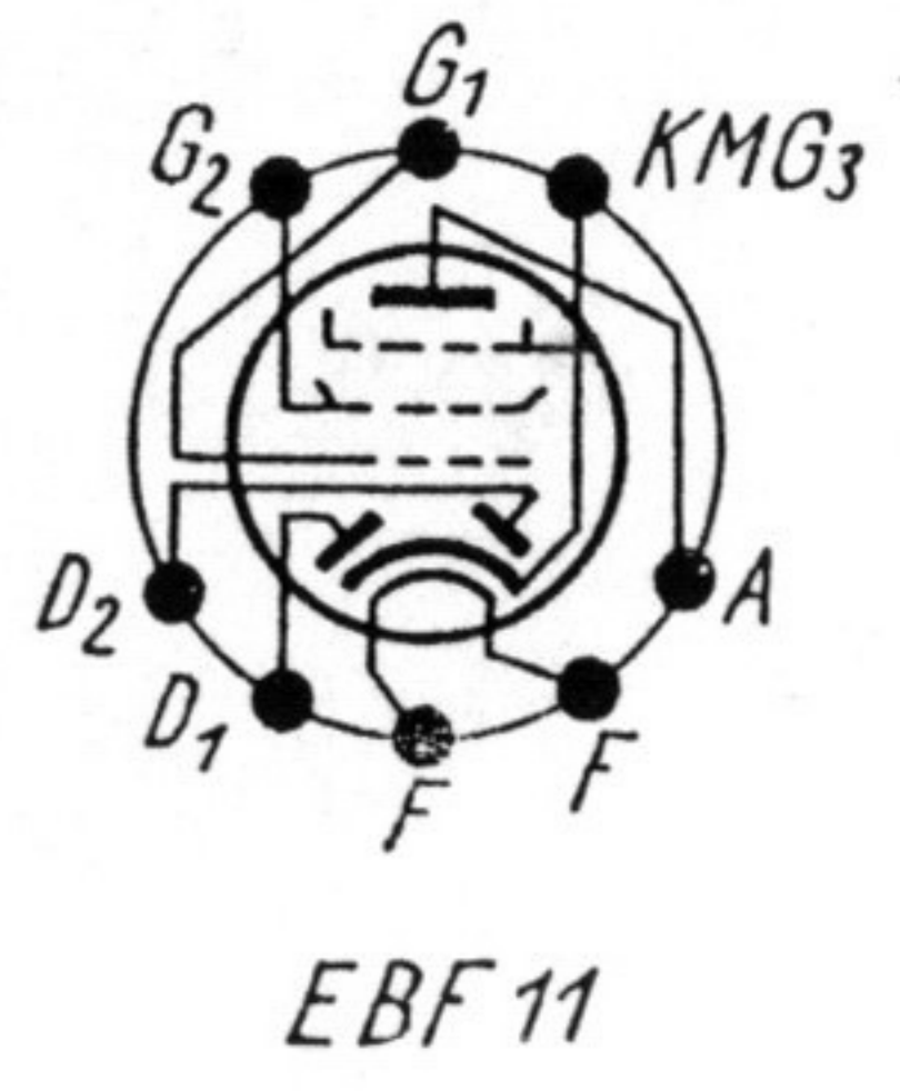
Röhrensockelschaltbilder (Sockel und Fassungen von unten gesehen)
