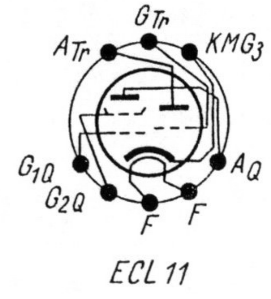
Röhrensockelschaltbilder (Sockel und Fassungen von unten gesehen)
