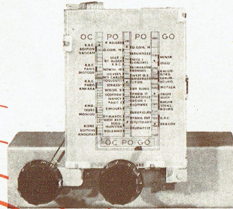
Réf. T 180. G/4249 A Visibilité 65×80 mm Cadran positif crème n° 582 OC - PO - GO
