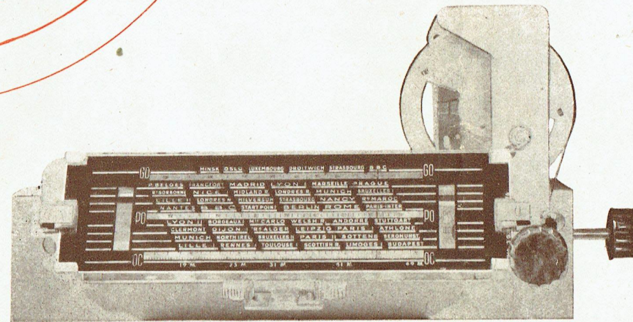
Réf. P 180. L/4249 A Visibilité 190×60 mm Cadran miroir n° 576 OC - PO - GO
