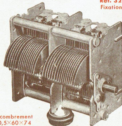
Réf. 3249 F Fixation 646
