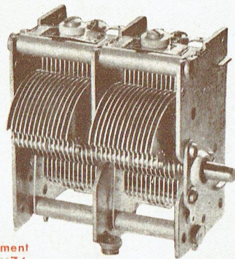
Réf. 3249 A Fixation 649
