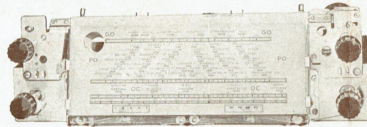
Réf. C 493. L Visibilité 360 à 390x110 mm Cadran positif crème n° 539 OCI - OC2 - PO - GO Cadran positif crème n° 550 OCI - OC2 - PO GO (Sécurité 615) Cadran positif crème n° 573 OC1 - OC2 - PO - GO (Visodion V. 204) Cadran positif crème n° 559 5 OC - 1 PO (Supers. Col. 63) Cadran positif crème n° 597 2 OC - 2 PO - GO (Artex 1520)
