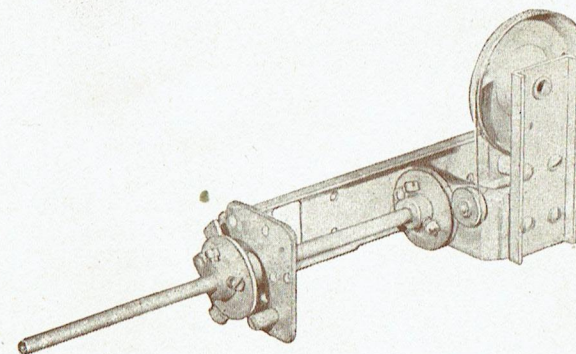
Commande perpendiculaire de contacteur Réf. n° 614 (commande à droite) Réf. n° 615 (commande à gauche)
