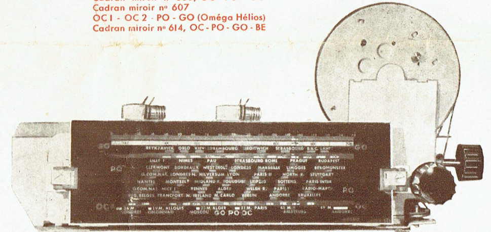
Réf. A 180. L Visibilité 201×60 mm Cadran positif n° 564 Cadran miroir n° 569 OC - PO - GO
