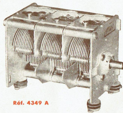
Encombrement 54x52x75
