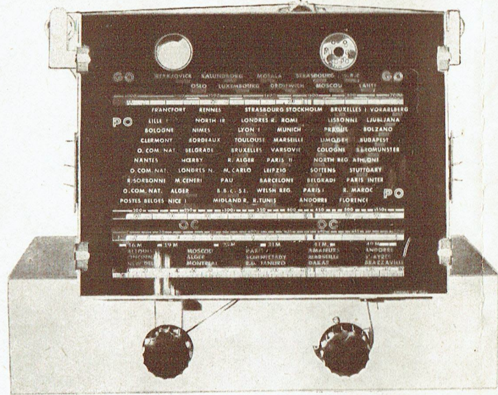
Réf. SR 183. G. (cadran droit) Visibilité 200×170 mm Cadran miroir n° 609, OC - PO - GO Cadran miroir n° 610, OC1 - OC2 - PO - GO Cadran miroir n° 611, OC1 - OC2 - OC3 - PO (Supers. Col. 42) Cadran miroir n° 612, OC1 - OC2 - PO - GO (Visodion V. 204) Cadran miroir n° 613, OC1 - OC2 - PO1 - PO2 GO (Artex 1520)
