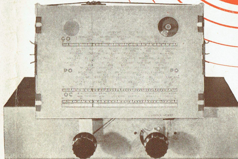
Réf. MRE 183. G/3249 A (cadran droit) Réf. MIRE 183. G/3249 A (cadran incliné) Visibilité 160×124 mm Cadran miroir n° 605 (sans œil) Cadran miroir n° 604 (avec œil) OC - PO - GO
