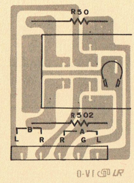
P.C.B., headphone-jack Platine prise-casque LTP Kopfhörerbuchse Platina toma auriculares Piastra presa per cuffia
