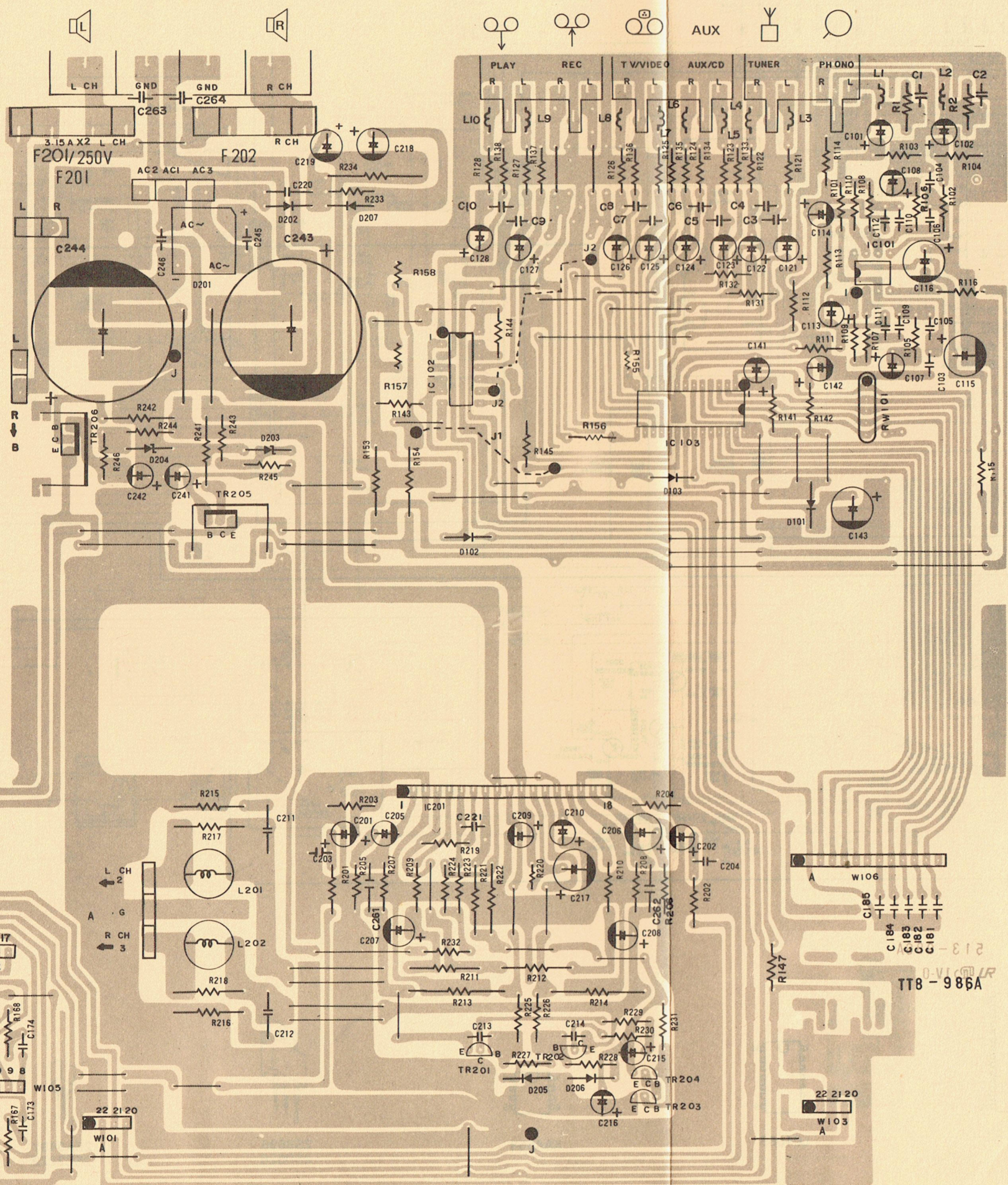
Main P.C.B. Platine principale Grundplatte Platina principal Piastra principale
