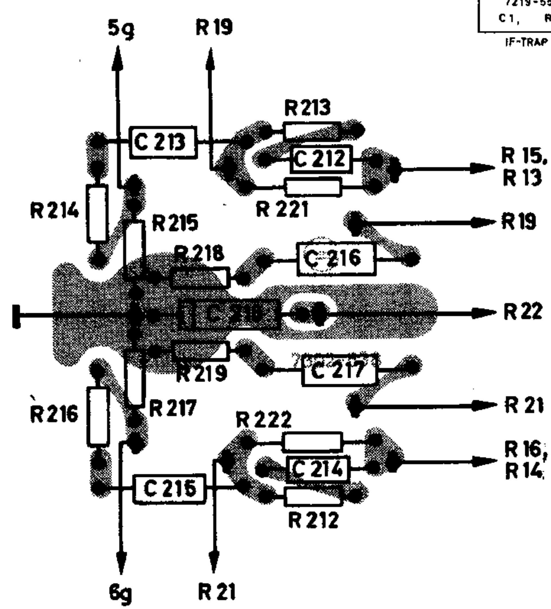
Potentiometerplatte HF 10, auf die Bestückungsseite gesehen
