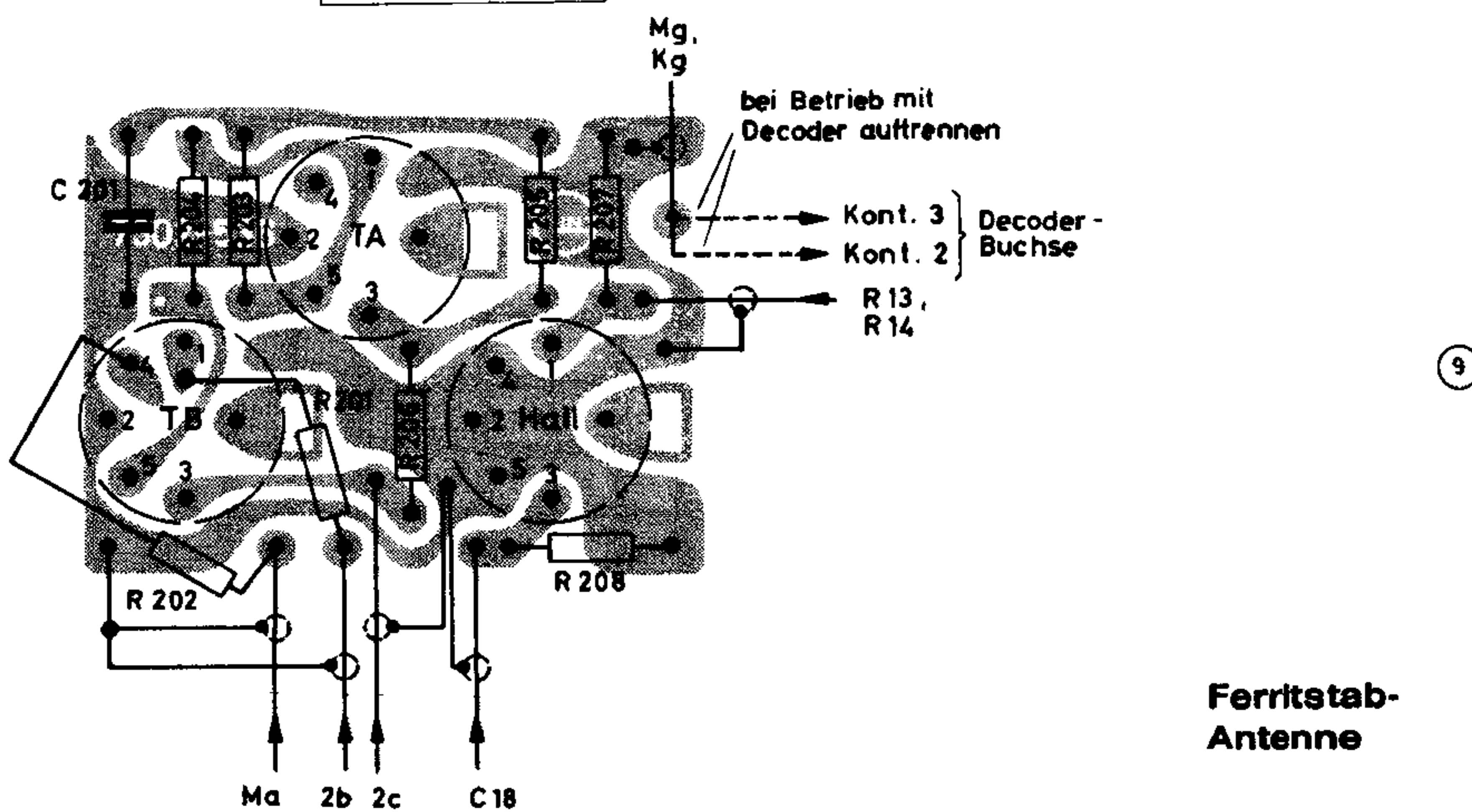
Anschlußplatte HF 10, auf die Lötseite gesehen
