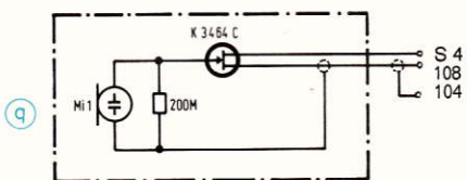
Schaltung des Electret-Mikrofons
