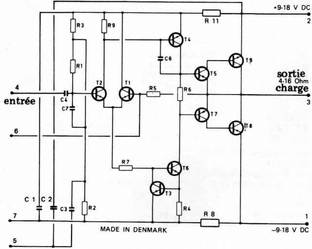
JOSTYKIT POWER AMPLIFIER AF 310-3
