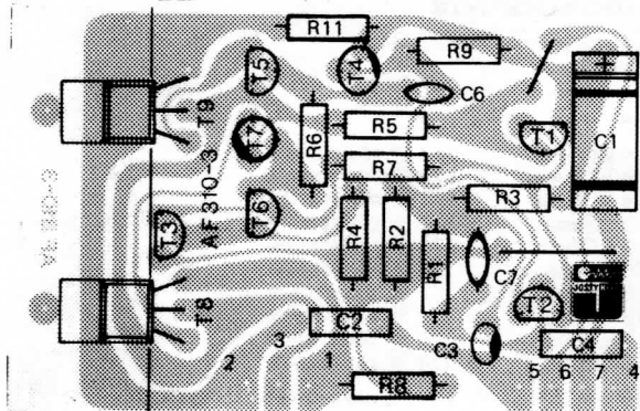
JOSTYKIT POWER AMPLIFIER AF 310-3
