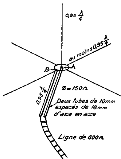
FIG. III-13. — Adaptation d'une antenne ground-plane à une ligne de 600 Ω.
