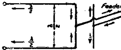
FIG. VI-20. — Mise en phase de deux éléments demi-onde alimentés au centre.
