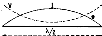
FIG. II-43. — Répartition de I et V dans une antenne demi-onde sans tenir compte des phases.
