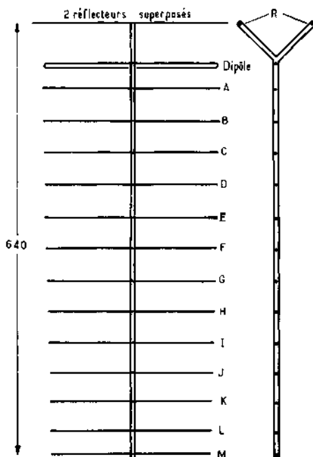
FIG. 53 c. — Antenne 16 éléments Tonna
