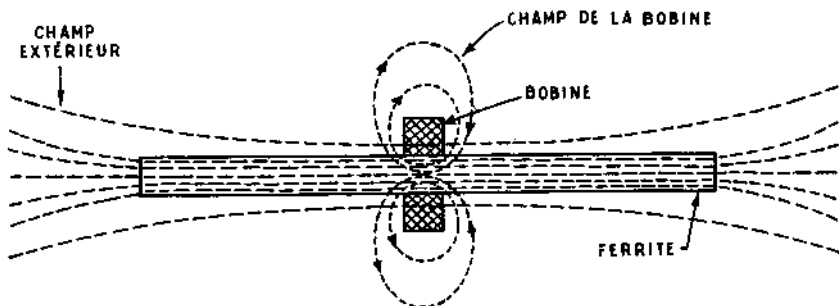
FIG. XI-4. — L'influence de la perméabilité du barreau est grande pour le champ de l'émetteur, mais elle est de peu d'importance dans l'augmentation de l'inductance du bobinage car les lignes de champ effectuent un parcours très réduit dans le barreau, la plus grande partie de ce parcours ayant lieu dans l'air.
