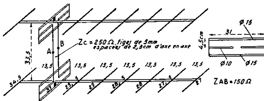
FIG. VI-40. — Antenne deux fots huit éléments pour 432 MHz. Gain : 16 dB environ. Écartement : 0,2\lambda entre éléments. Éléments en tige de 5 mm. Espacement \lambda/2 .
