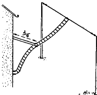
FIG. II-23. — Soutien d'une ligne à fil parallèles par une ligne fermée \frac{\lambda}{4} . L'isolement n'existe que pour la longueur d'onde \lambda . Pour une longueur d'onde moitié la ligne de soutien devient un court-circuit.
