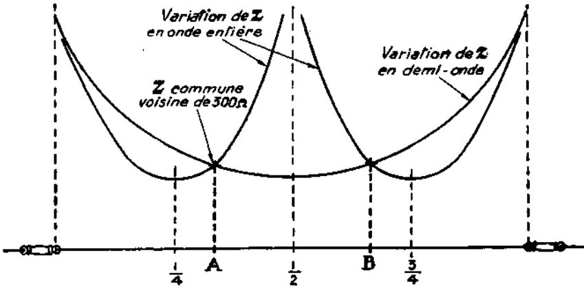
FIG. III-23. - A et B : points d'attache de l'antenne demi-onde ou onde entière.
