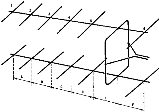
FIG. VI-83. Antenne 435 Yagi avec radiateur squelette 2 : 7 éléments.
