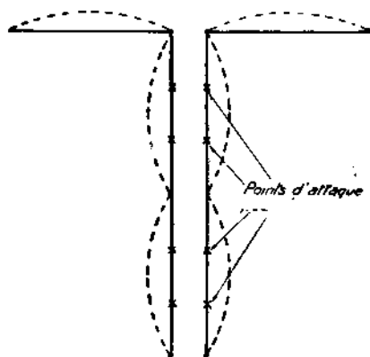
FIG. III-65. — Fonctionnement sur harmonique 2 dans la bande 40 m. Attaque par ligne de 300 Ω.
