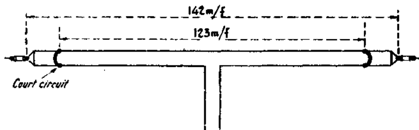
FIG. III-38. Antenne pliée réalisée en twin-lead 300 Ω et court-circuitée aux extrémités (voir texte).
