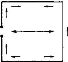
FIG. VI-64 a. — Antenne carrée alimentée sur le côté
