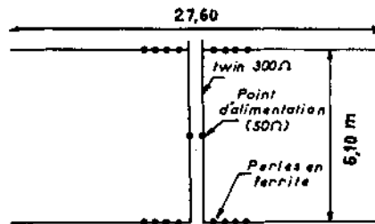
Fig. VI-112. Superpositions de deux antennes F.B.5.
