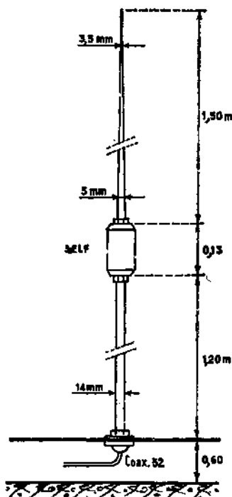
FIG. VII-2. — Schéma général
