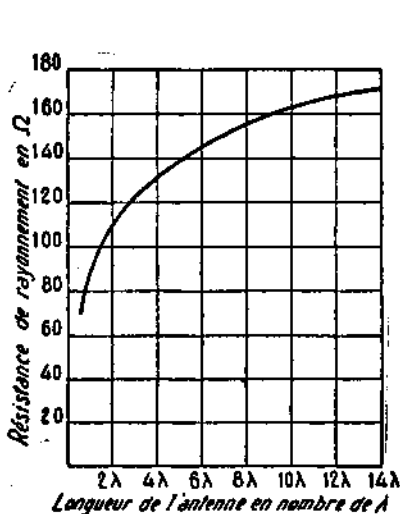
FIG. II-48. — Résistance de rayonnement en fonction de la longueur de l'antenne supposée en résonance.
