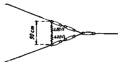
FIG. VI-10. — Dessin donnant la façon de brancher les résistances terminales.
