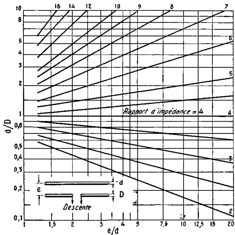
FIG. 5H-29. — Abaque donnant le facteur multiplicateur d'impédance dans un trombone à 2 éléments de diamètres différents.
