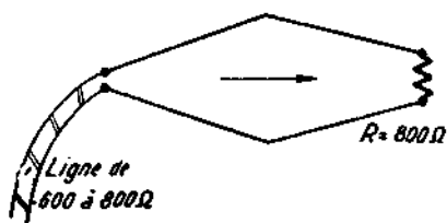
FIG. VI-9. — Antenne losange aperiodique et unidirectionnelle.
