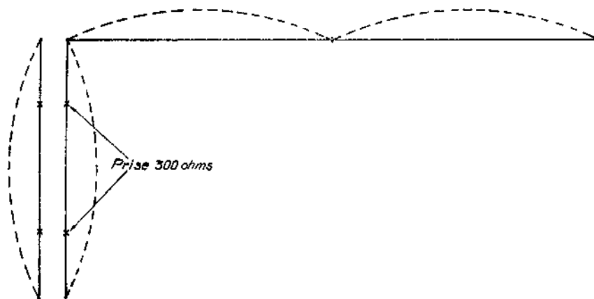
FIG. III-71. — Sur la bande 10 m, il y a deux emplacements possibles pour la prise de la ligne de 300 ohms
