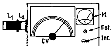
FIG. VIII-26. — Dispositif pratique.
