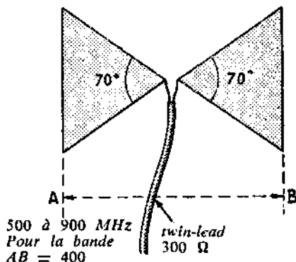
FIG. VI-77. Antenne drapeau. Gain de 1 à 4 dB (1 à 500 MHz, 4 à 900 MHz).
