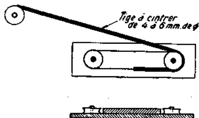
FIG. III-33. — Gabarit pour cintrer de la tige pletne d'aluminium ou de duralinox.
