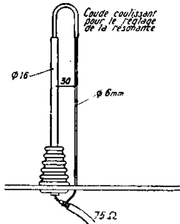
Fig. III-15. — Détails de fixation du demi-trombone.
