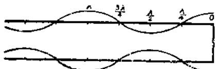
FIG. II-12. — Répartition réelle du courant dans une ligne fermée
