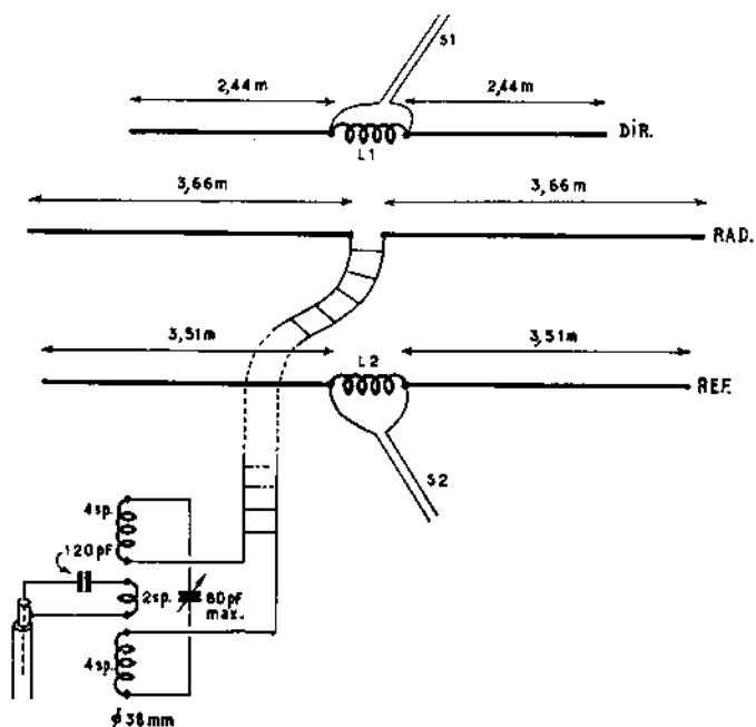
FIG. VI-110. --- La Mini-beam G4ZU.
