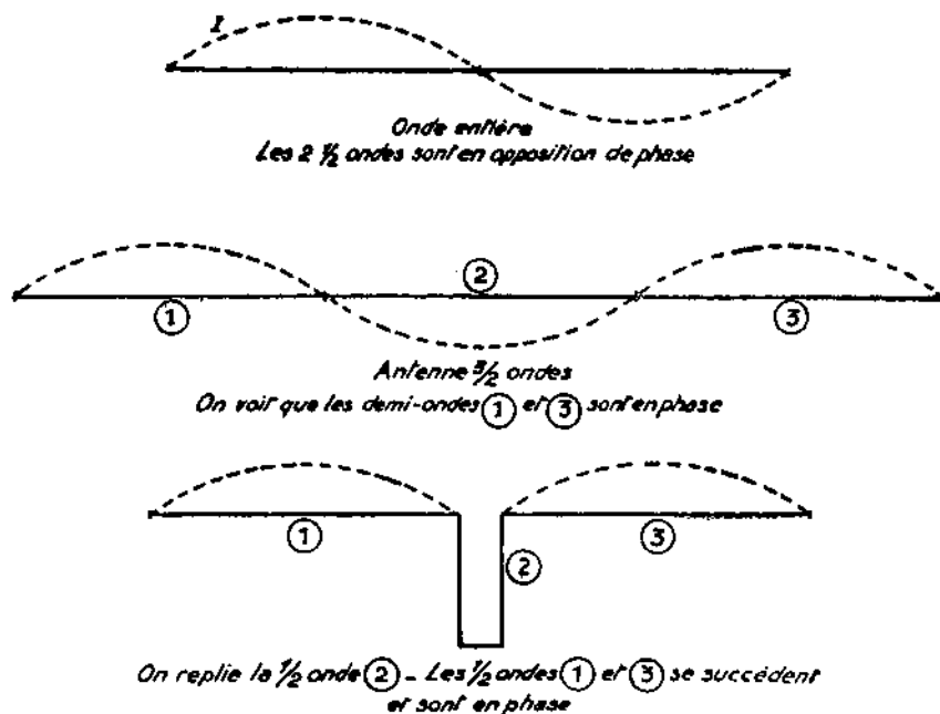
FIG. VI-12. — Antenne onde entière, antenne trois demi-ondes et transformation de celle-ci.
