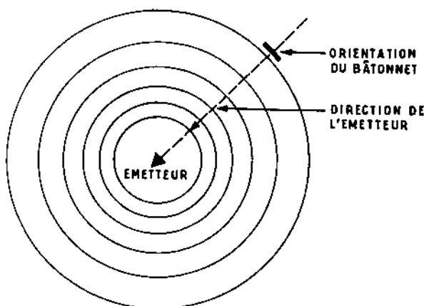
FIG. XI-5. — Le barreau doit être orienté perpendiculairement à la direction de l'émetteur pour être parallèle aux lignes de champ.
