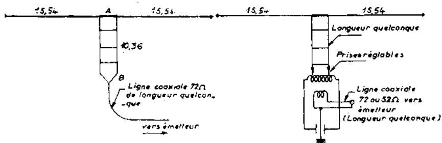
FIG. III-78 a. — FIG. III-78 b. — Deux systèmes d'alimentation possibles.
