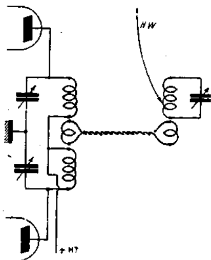
FIG. IX-5. — Couplage indirect d'une antenne Herix-Windom à un étage final push-pull.
