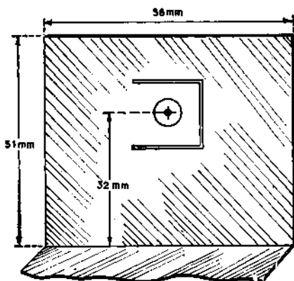
FIG. VIII-7 a. — Assemblée de la gouttière.
