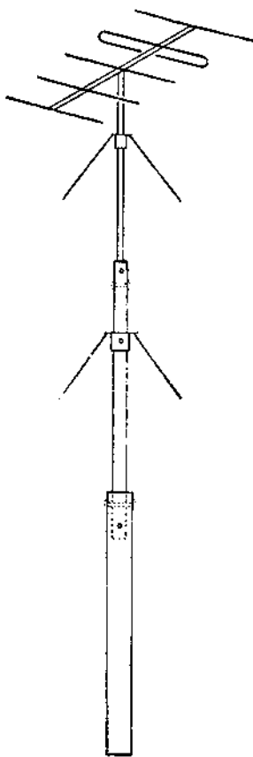
FIG. XI-5. — Mât fait de plusieurs tubes qui s'emboîtent.
