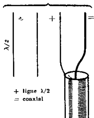
FIG. III-61. — Si le feeder a une longueur égale à une demi-onde, on peut l'attaquer avec un coaxial dont l'impédance est égale à l'impédance au centre de l'antenne.
