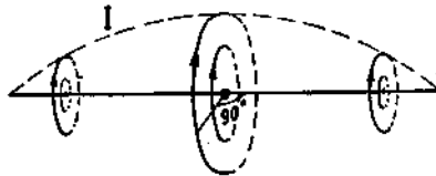
FIG. 11-40. — Champ magnétique créé par le courant dans l'antenne \frac{\lambda}{2} . Aux extrémités I est nul, le champ est nul ; au milieu I est maximum : le champ est maximum. Le plan des lignes de force est perpendiculaire à l'antenne.
