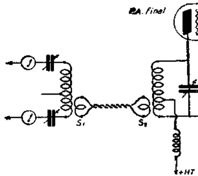
FIG. III-55 b. — Couplage direct d'une ligne à ondes stationnaires. S_1 et S_2 comportent chacune 2 ou 3 spires, couplées du côté froid, c'est-à-dire au milieu de la self d'antenne pour S_1 et du côté haute tension pour S_2 . Le fil torsadé peut avoir une longueur quelconque.
