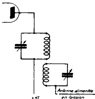
FIG. IX-11. — Couplage d'une antenne alimentée en tension à un étage final antique.
