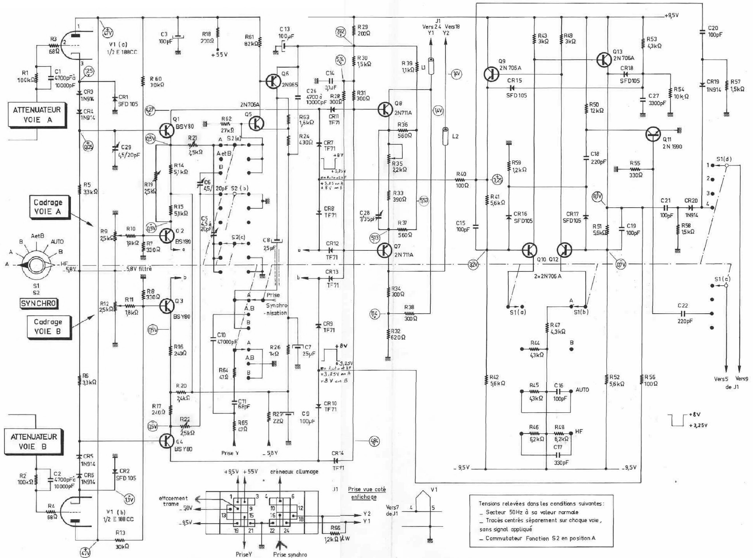
Planche 2.5 : TIROIR COMMUTATEUR ELECTRONIQUE
