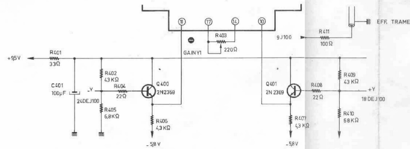
Planche 2.2 : AMPLIFICATEUR VERTICAL
