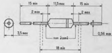
SOD 35
