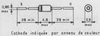
D0 41
