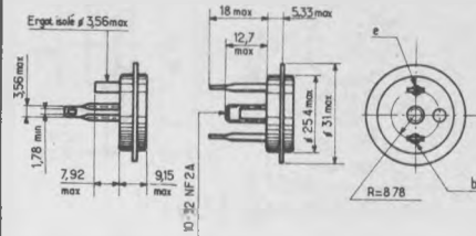
TO 39(A) Emetteur au boîtier
