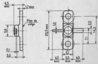
F0 41
