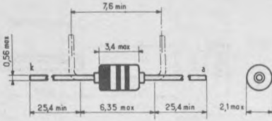
SOD 17
