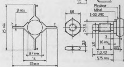
SOT 55/3
