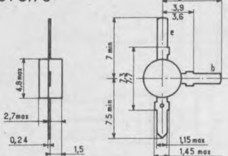
SOT 48/2
