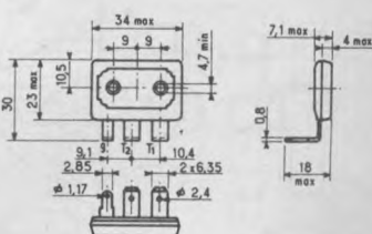
SOT 80
