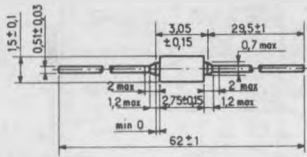
D0 41
