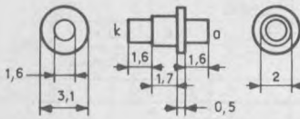
SOD 34 (1)
