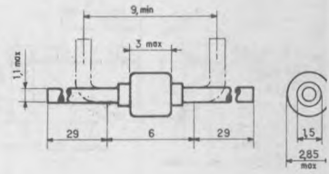
SOD 56
