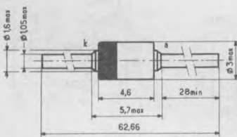
SOD 57
