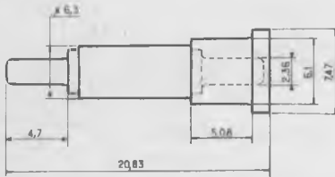
D0 34
