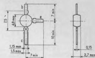
SOT 42
