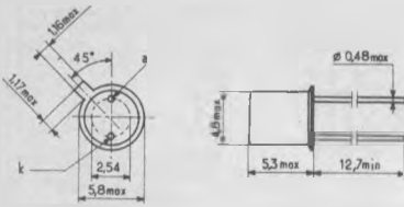
TO 18 modifié
