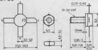
SOT 56
