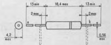
SOD 59
