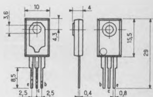
TO 66 plastique ( TO 220 ancienne version )
