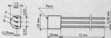
SOT 42
