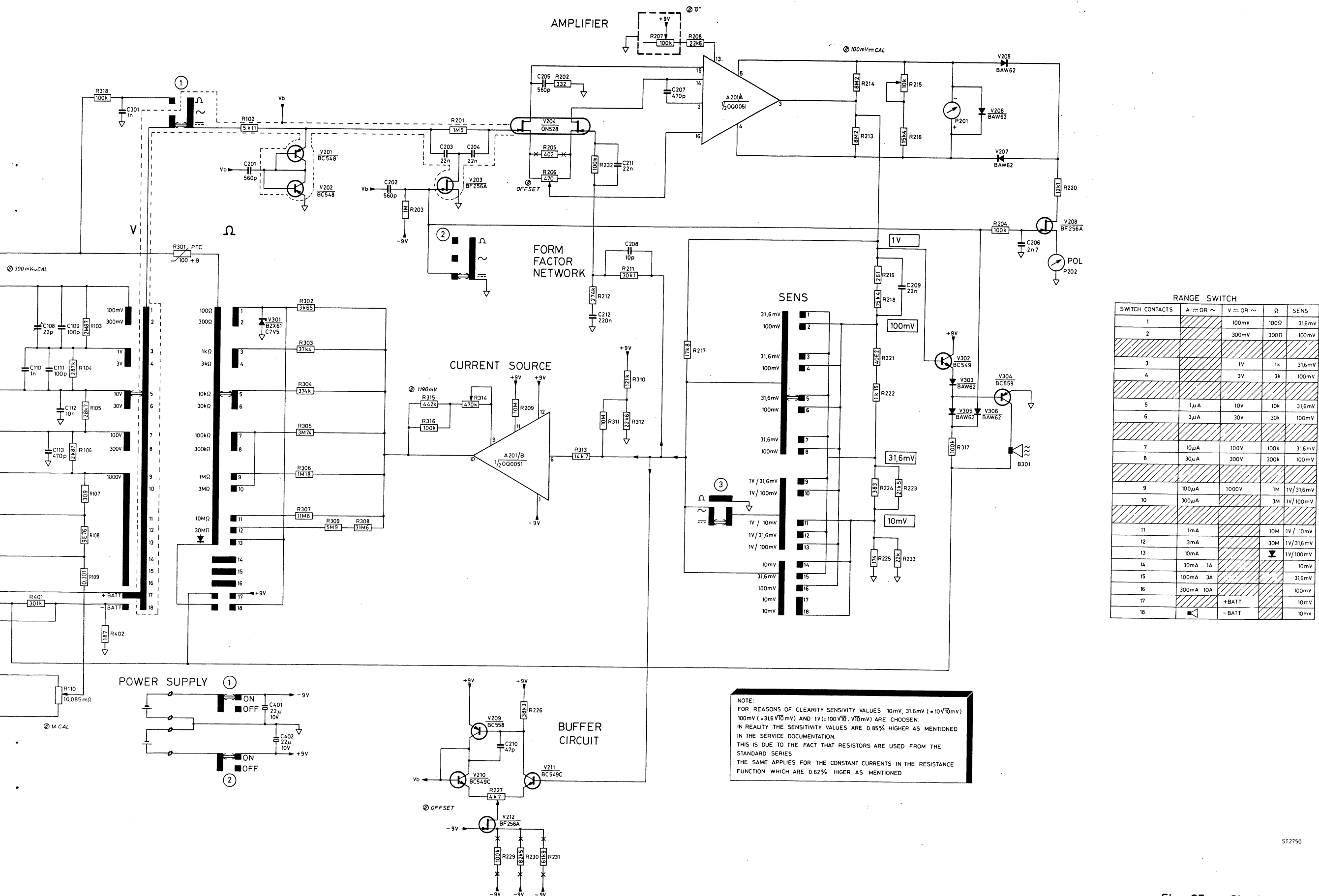
Fig. 25. Circuit diagram
