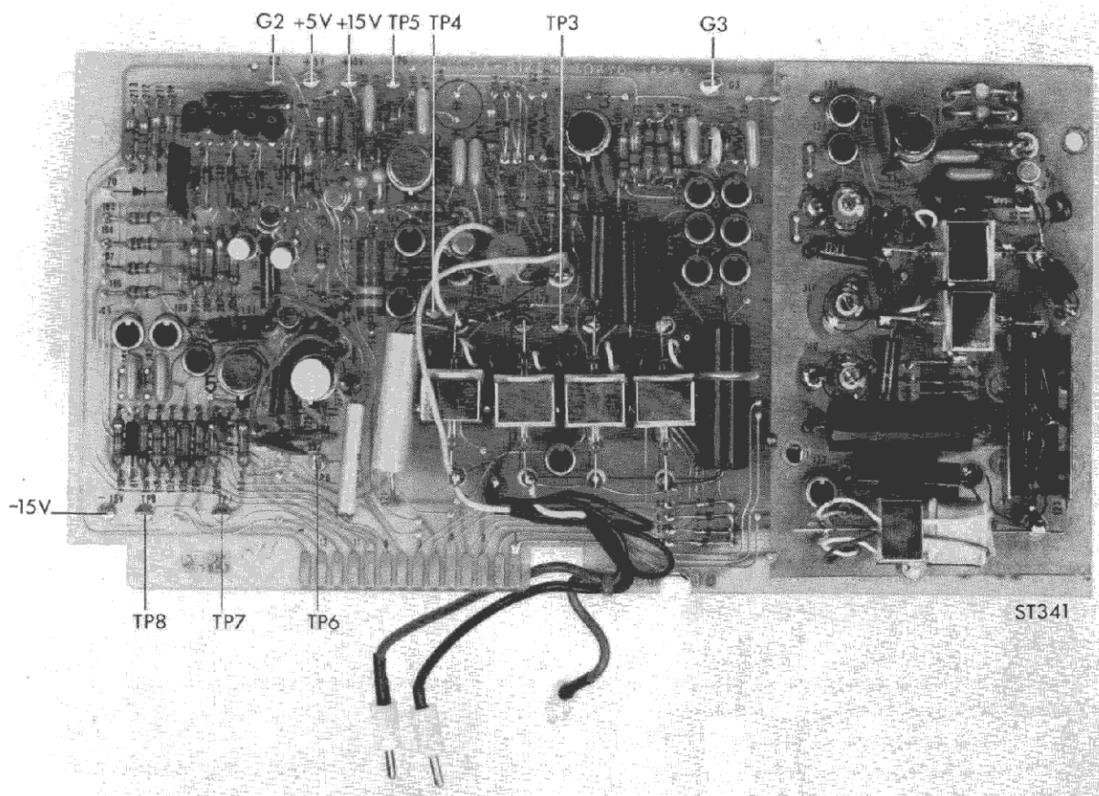
Fig. 27. Test points on unit U1
