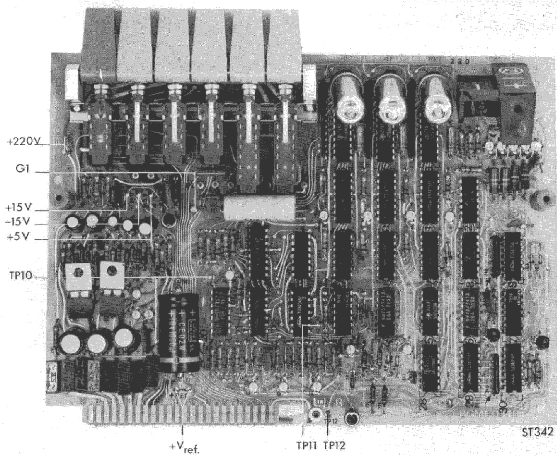
Fig. 28. Test points on unit U2
