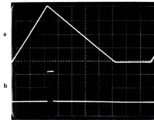
Fig. 24. Down signal
