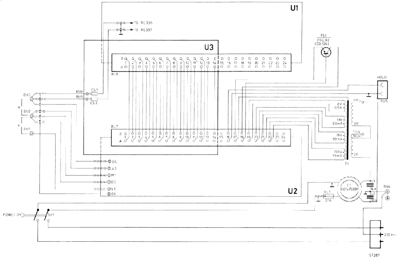
Fig. 36. Wiring diagram
