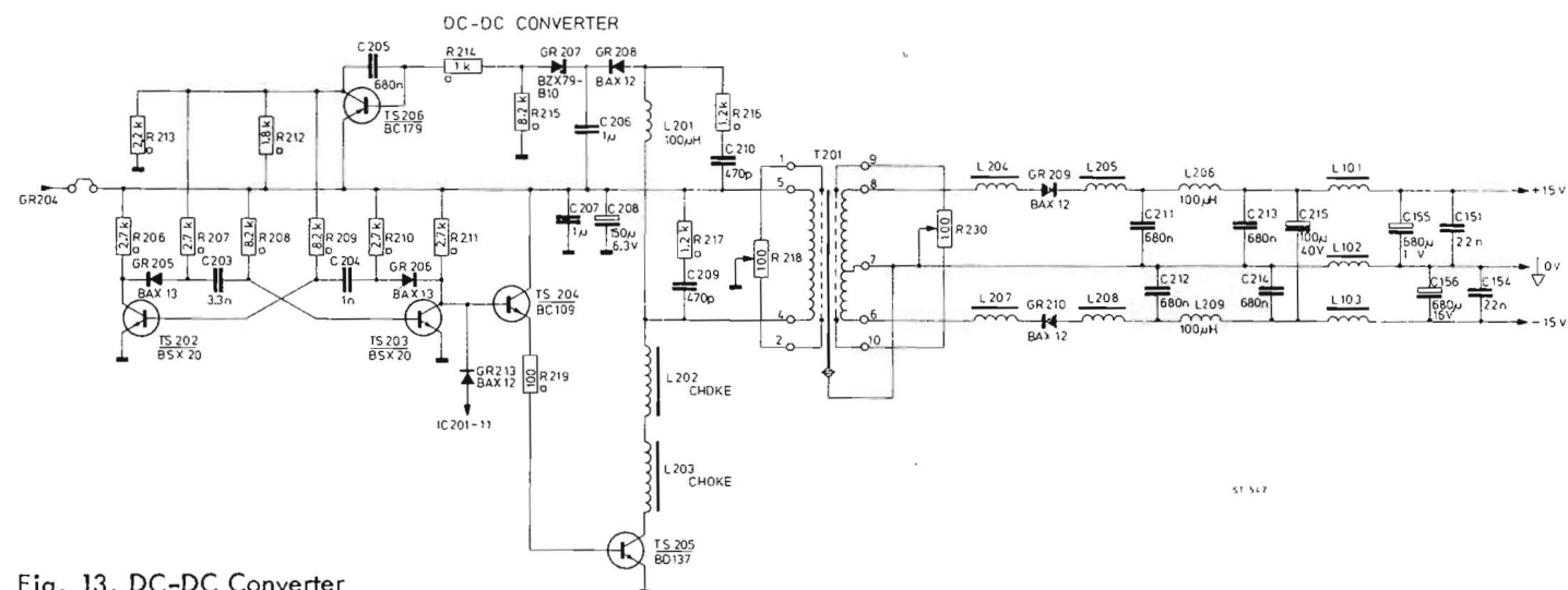
Fig. 13. DC-DC Converter
