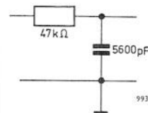
Fig. 8. Laagdoorlaatfilter
