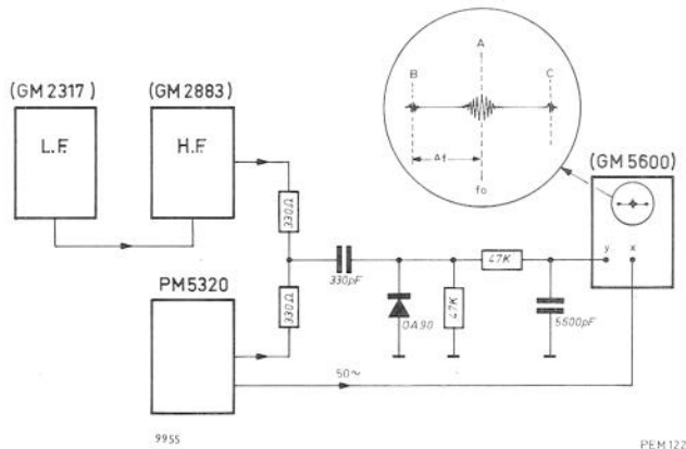
Fig. 35. Schakeling voor het meten van de frequentiezwaaai
