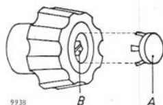
Fig. 30. Verwijderen van de knoppen
