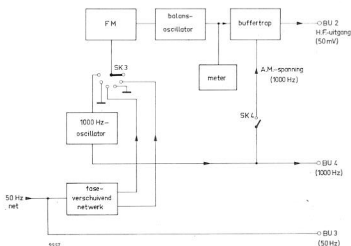
Fig. 1. Blokschema
