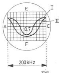
Fig. 23. M.F.-kromme in twee stadia van afregeling
