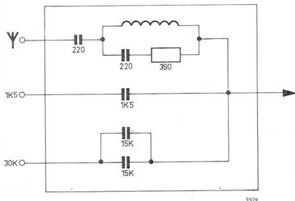
Fig. 4. Schema van de kunstantenne PM 9532 N
