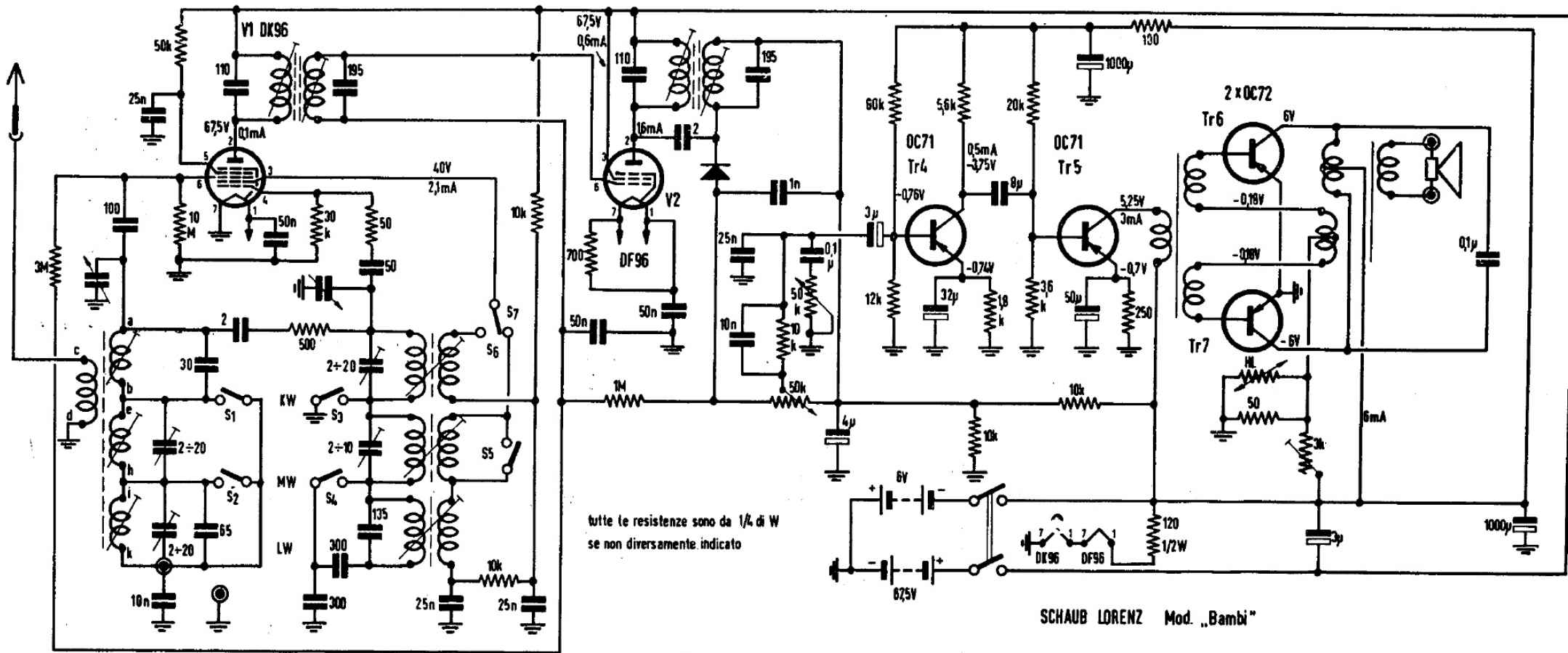
Schema elettrico del radiorecettore SCHAUB LORENZ mod. Bambi
