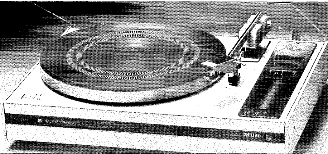
GA 209 S électronique automatique. 3 moteurs indépendants, asservissement tachymétrique, cellule "Super M" GP 412 VE. Prix : 1795 F*
