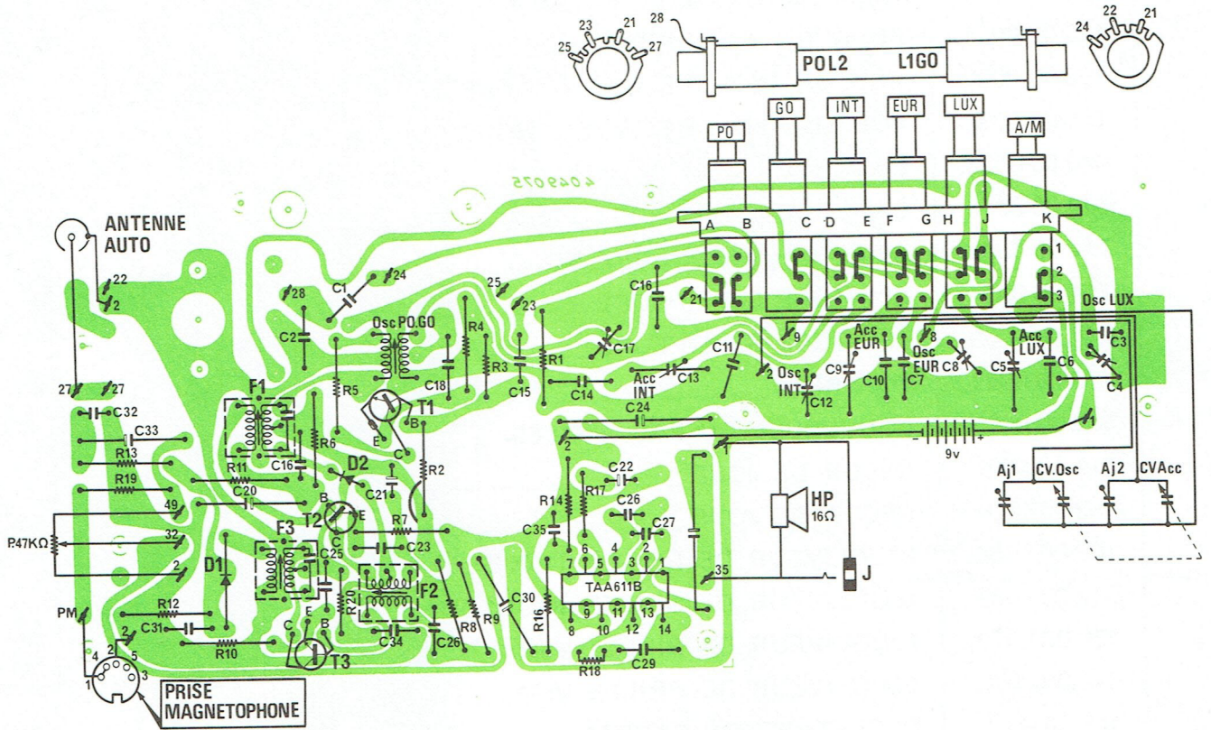
CIRCUIT IMPRIMÉ VU COTÉ ÉLÉMENTS
