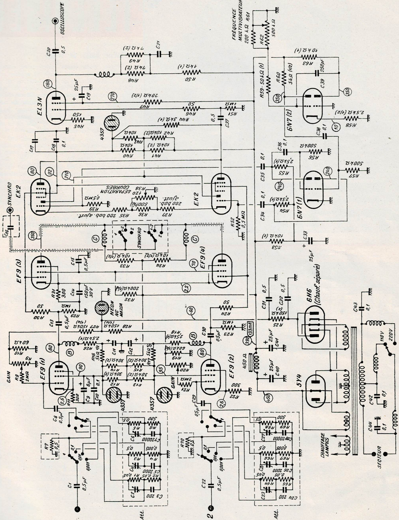
Schéma général du Commutateur Electronique 715 B. Les condensateurs découplant l'écran de la EF 9 (2) à la masse ont été oubliés : 8 \mu F et 0,1 \mu F en parallèle.
