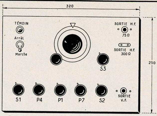
DISPOSITION DE LA FACE AVANT
