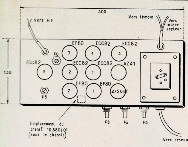
DISPOSITION DU CHÂSSIS
