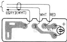
【NEON LAMP BOARD】 (CONDUCTOR SIDE)
