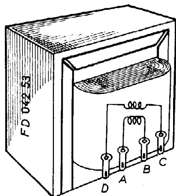
Transformateur de HP
