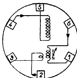
Découplage antenne
