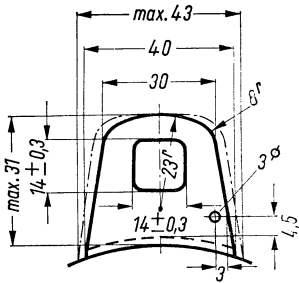
Einzelheit „C“
