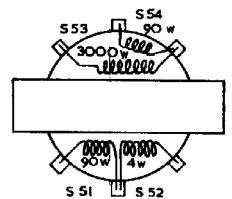
UITGANGSTRAFO GK 512 80
