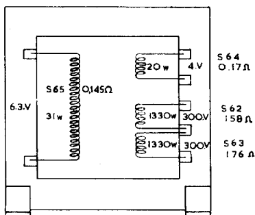
VOEDINGSTRAFO GK 512 74
