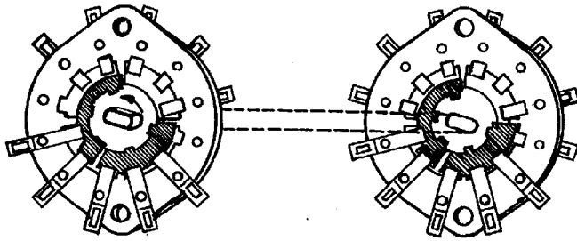
DE TWEE SEGMENTEN VAN DE GOLFBEREIKSCHAKELAAR NAAR DE KNOP TOE GEZIEN
