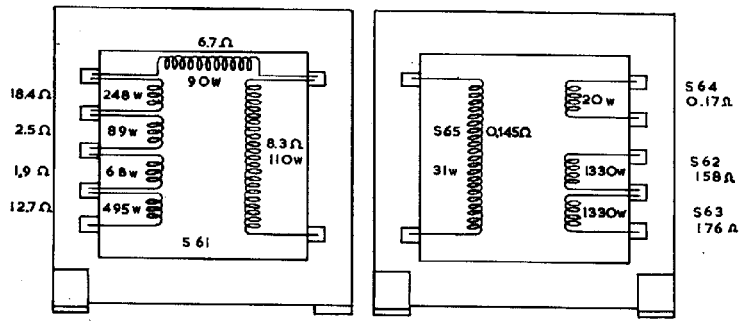
VOEDINGSTRAFO GK 512 74
