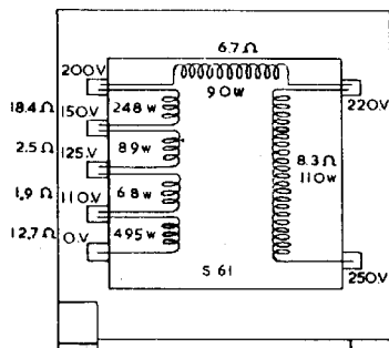
VOEDINGSTRAFO GK 512 74
