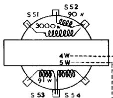
UITGANGSTRAFO GK 512 90 KY 505N 506N GK 512 80 KY 505 506
