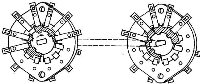
DE TWEE SEGMENTEN VAN DE GOLFBEREIKSCHAKELAAR VANAF DE KNOP GEZIEN
