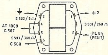
RASTER UITGANGS TRAFU FRAME OUTPUT TRANSF. BILDAUSG. ÜBERTRAGER AT 3502
