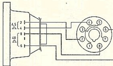
DEFLECTIE JUK DEFLECTION YOKE ABLENKEINHEIT AT 1009
