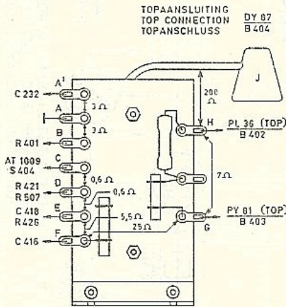
LIJNUITGANGS TRAFU LINE OUTPUT TRANSF. ZEILENAUSG. ÜBERTRAGER AT 2018/20
