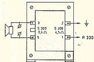
GELUID UITGANGS TRAFU SOUND OUTPUT TRANSF. TONAUSG. ÜBERTRAGER GK 515 81
