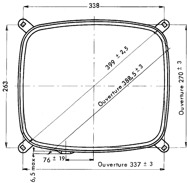
ENCOMBREMENT (cotes en mm)
